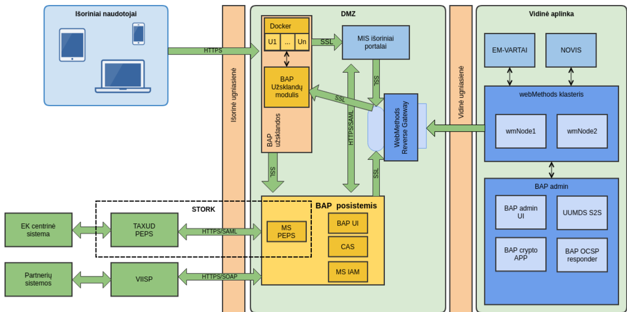
8 pav. Detali BAP architektūra
