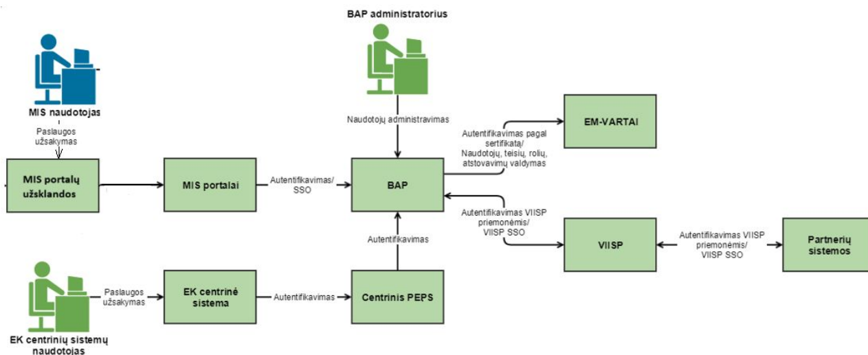
6 pav. Principinė BAP veiklos architektūra
