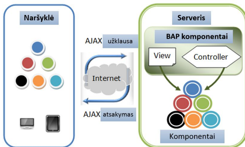
7 pav. supaprastinta ZKoss karkaso architektūra
