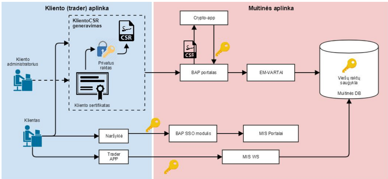
9 pav. Muičinės sertifikatų išdavimo schema
