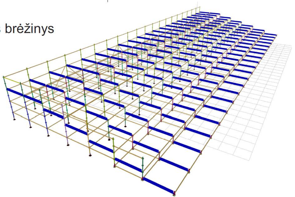
Pav. 4.1 Tribūnos konstrukcijos brėžinys
