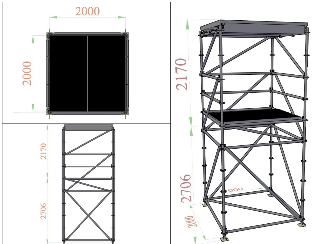
Pav. 1.3. Projekcinio bokštelio matmenys
