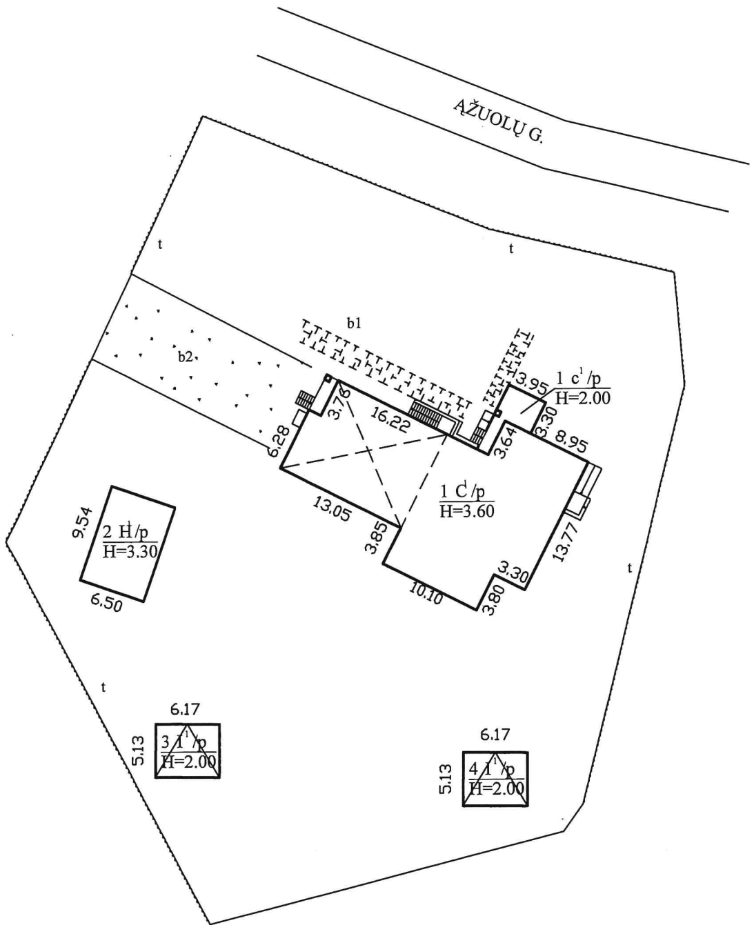
Statinių išdėstymo planas sudarytas pagal 2011 m. UAB "EVII" parengtą žemės sklypo planą.
