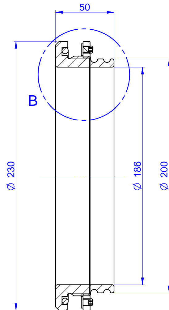
SECTION A-A
