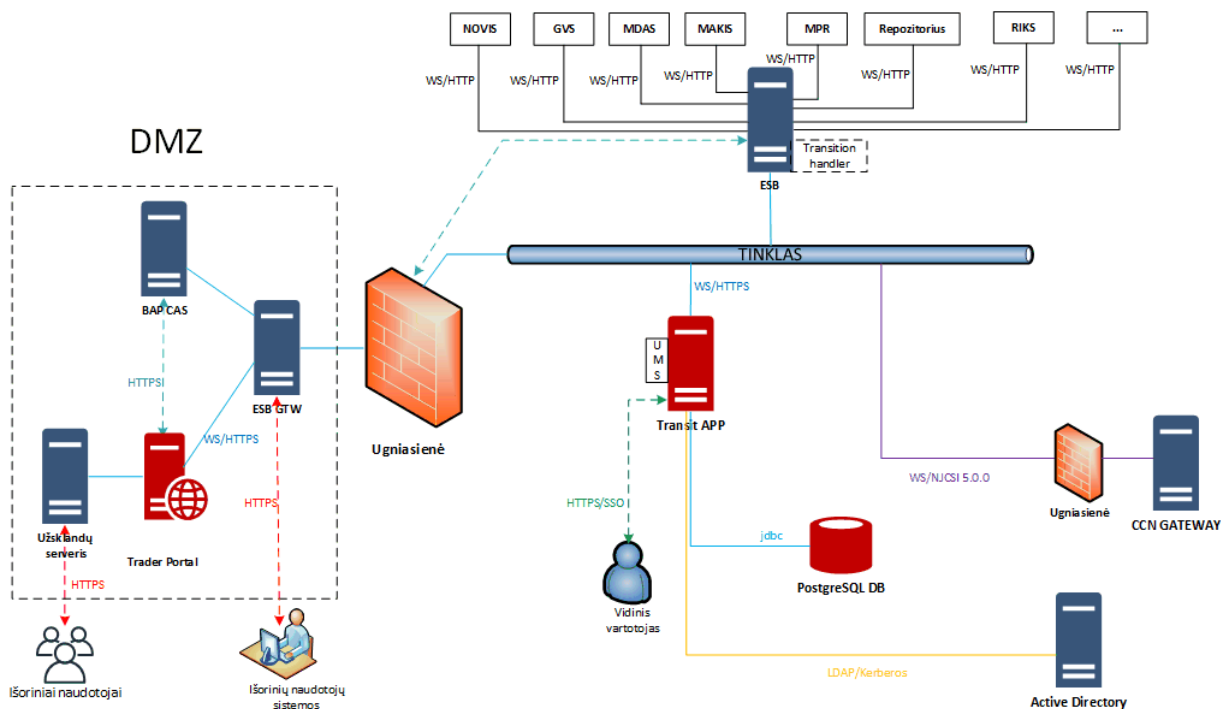
8 pav. NTKS architektūrinis sprendimas
