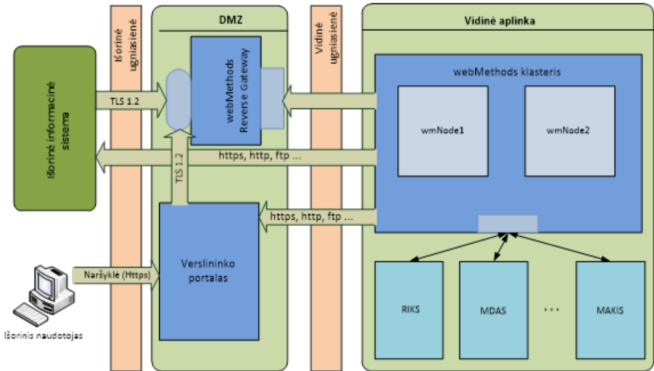
4 pav. Sąveikos su išorinėmis sistemomis principinė schema
