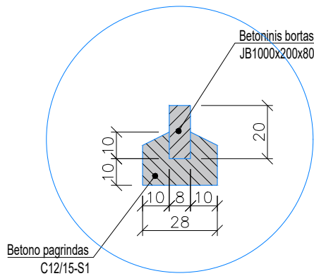
Detalé M1:20
