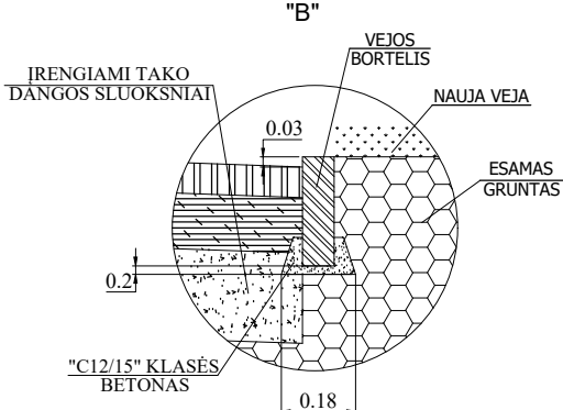
VEJOS BORTELIO ĮRENGIMO MAZGAS
