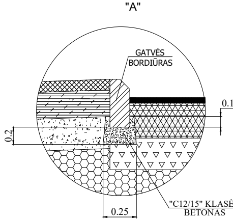
GATVĖS BORTO ĮRENGIMO MAZGAS
