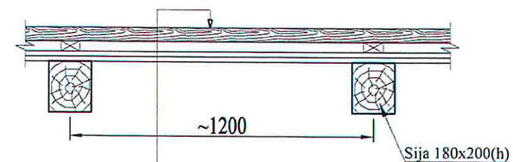
Pirmo aukšto perdangos detalė "C" M 1:20
