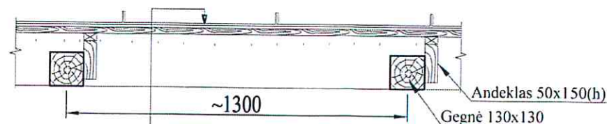
Stogo detalė "F" M 1:20
