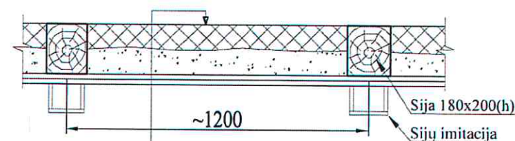
Perdangos virš mansardos detalė "E" M 1:20
