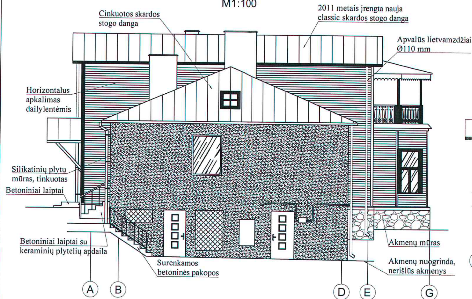
FASADAS TARP AŠIŲ A-G M1:100
