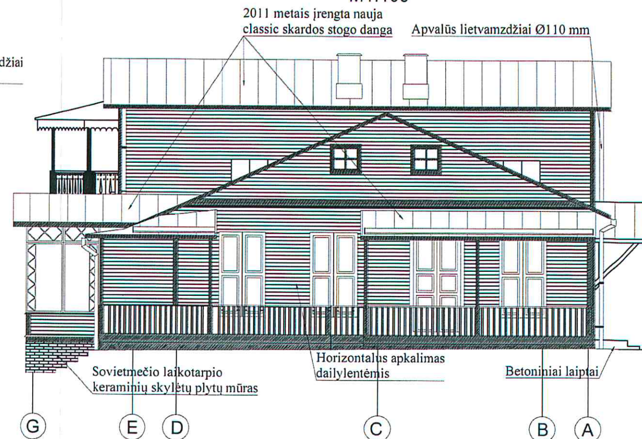
FASADAS TARP AŠIŲ G-A M1:100
