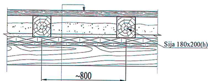
Pirmo aukšto perdangos detalė "D" M 1:20
