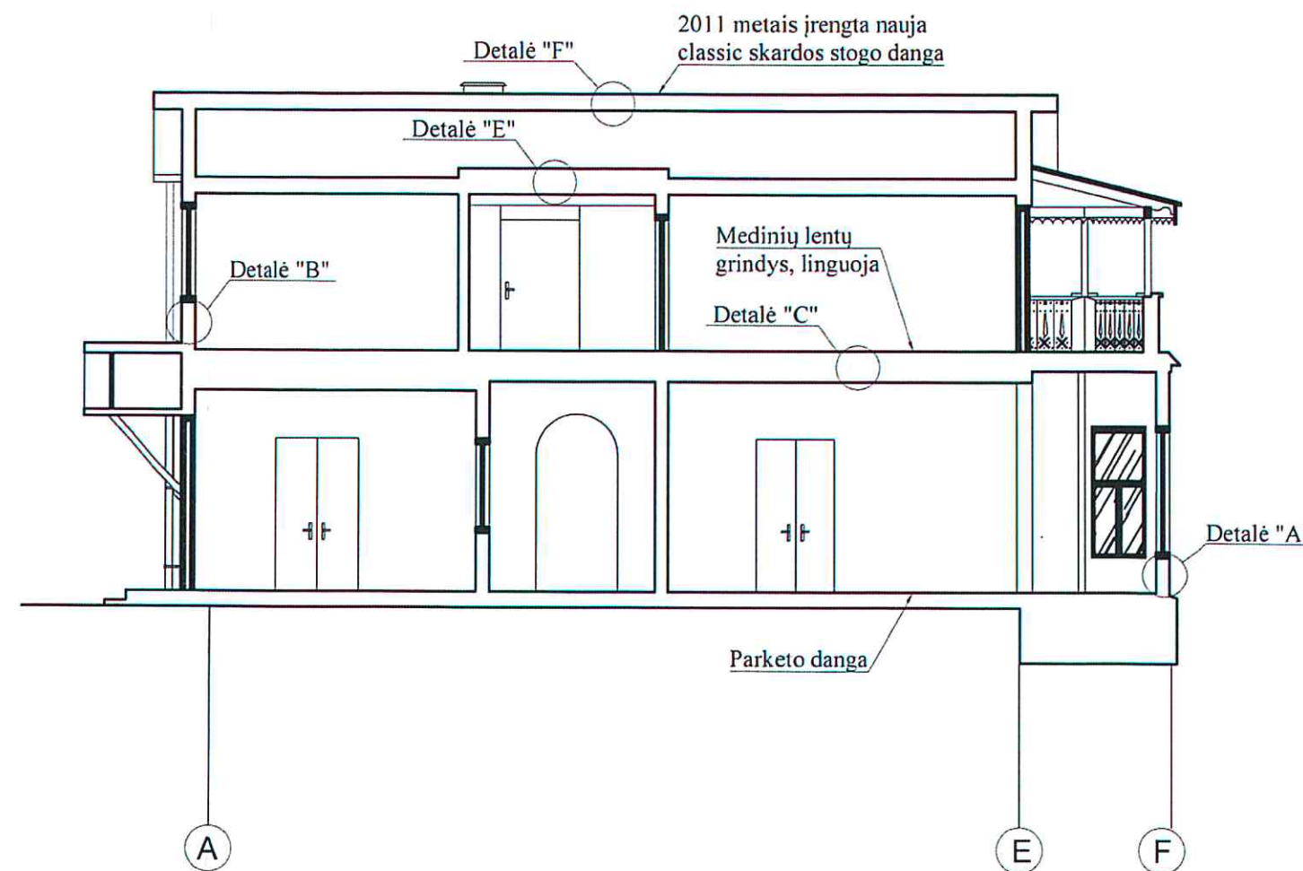
PJŪVIS 2-2 M1:100
