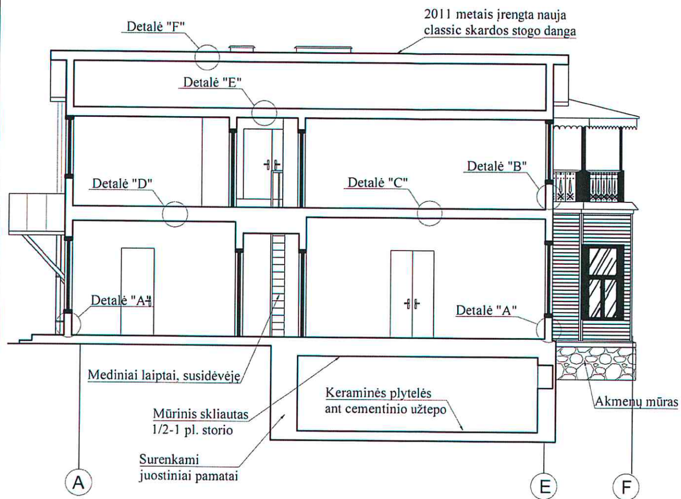
PJŪVIS 3-3 M1:100
