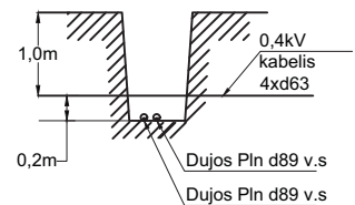
SUSIKIRTIMAS SU ESO TINKLAIS SKERSINIS PJŪVIS LE1-5
