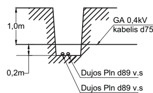
SUSIKIRTIMAS SU DUJŲ TINKLAIS SKERSINIS PJŪVIS LE3-15
