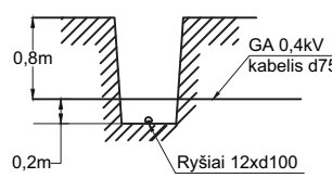
SUSIKIRTIMAS SU RYŠIŲ TINKLAIS SKERSINIS PJŪVIS LE3-13
