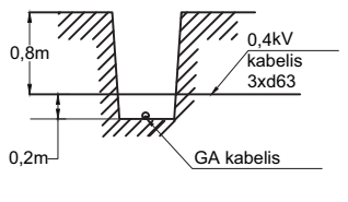
SUSIKIRTIMAS SU GA TINKLAIS SKERSINIS PJŪVIS LE1-7
