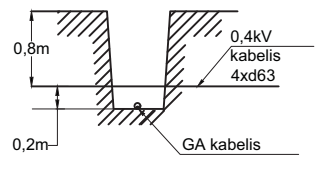
SUSIKIRTIMAS SU GA TINKLAIS SKERSINIS PJŪVIS LE1-5
