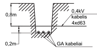
SUSIKIRTIMAS SU DUJŲ TINKLAIS SKERSINIS PJŪVIS LE1-11
