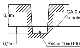
SUSIKIRTIMAS SU RYŠIŲ TINKLAIS SKERSINIS PJŪVIS LE3-3
