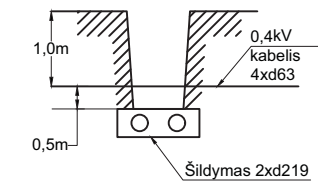
SUSIKIRTIMAS SU ŠILDYMO TINKLAIS SKERSINIS PJŪVIS LE1-8
