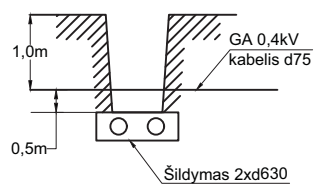
SUSIKIRTIMAS SU ŠILDYMO TINKLAIS SKERSINIS PJŪVIS LE3-18
