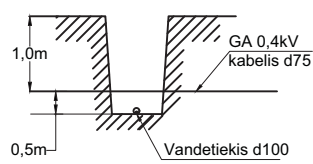
SUSIKIRTIMAS SU VANDENTIEKIO TINKLAIS SKERSINIS PJŪVIS LE3-12
