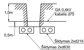
SUSIKIRTIMAS SU ŠILDYMO TINKLAIS SKERSINIS PJŪVIS LE3-16
