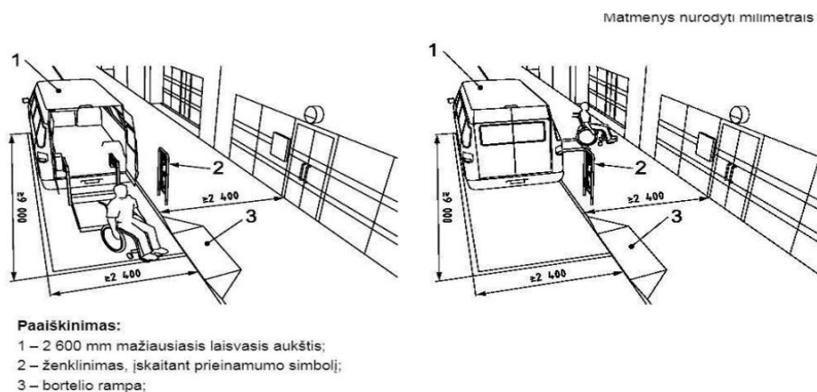
2 paveikslas. Išilgai šaligatvio įrengtos stovėjimo vietos pavyzdys
