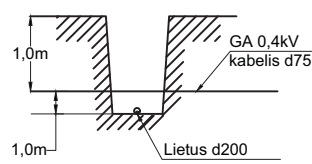
SUSIKIRTIMAS SU LIETAUS TINKLAIS SKERSINIS PJŪVIS LE3-14
