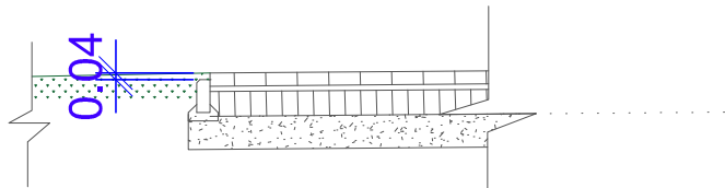
PASLĖPTO BORTO DETALĖ
