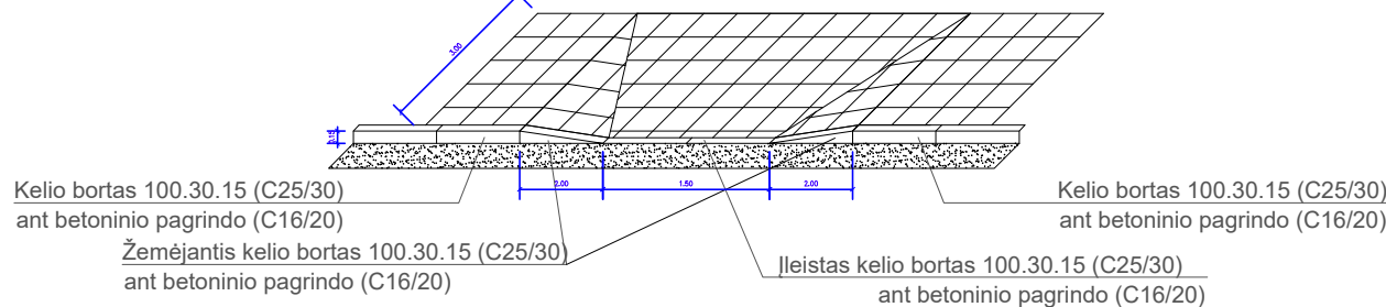
DETALĖ "B"(pandusas)
