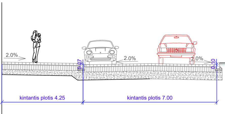
PJŪVIS C-C M 1:100
