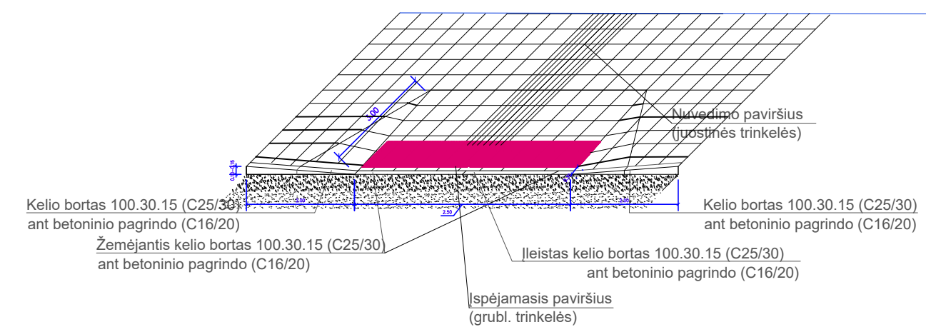
DETALĖ "A"(pandusas)
