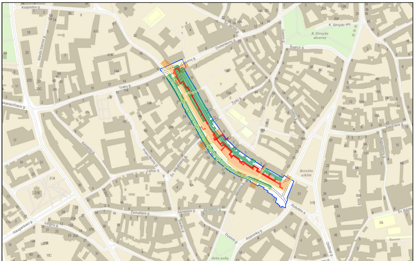
Situacijos schema 1:500
