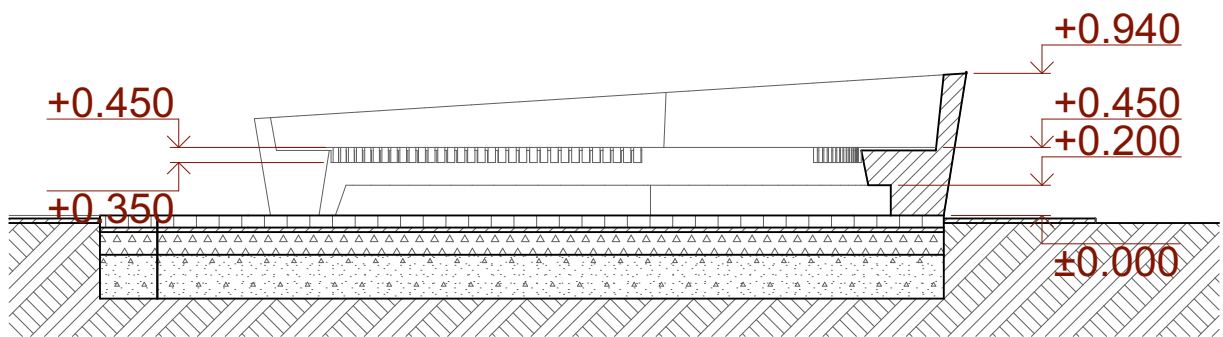
Pjūvis 3.1
