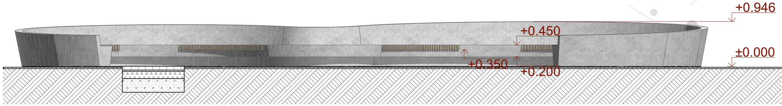
Fasado išklotinė 1.3
