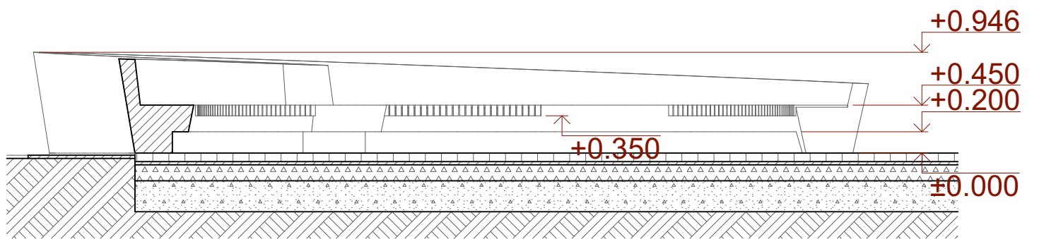
Pjūvis 1.3
