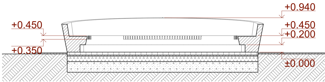
Pjūvis 3.2
