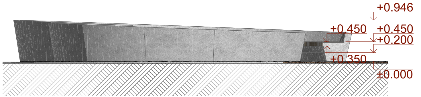
Fasado išklotinė 1.4
