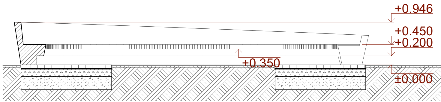
Pjūvis 1.2
