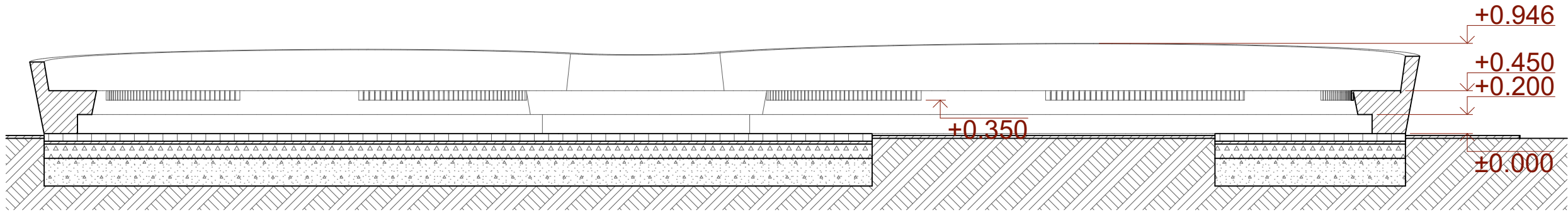
Pjūvis 1.1
