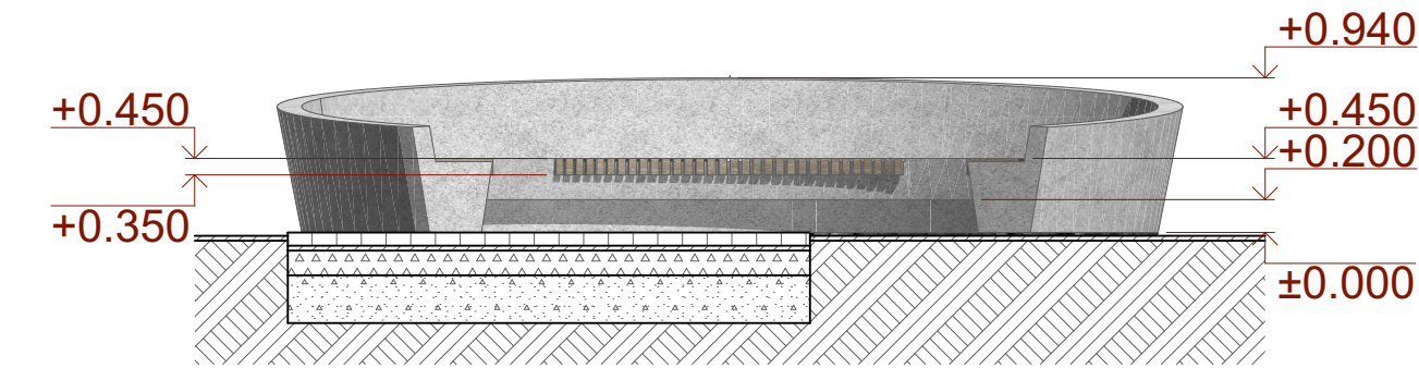
Fasado išklotinė 3.4
