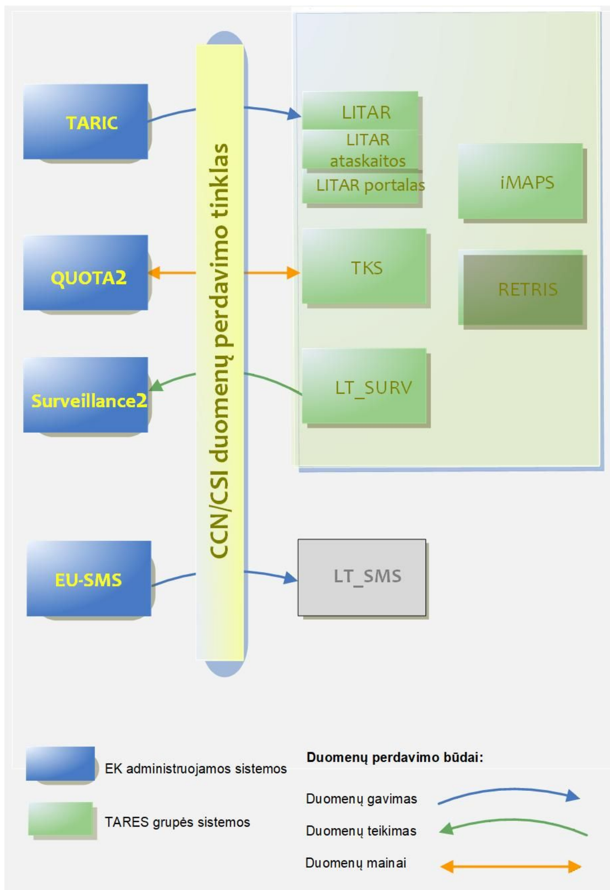
8 pav. TARES ir LT-SMS sąsajos su išorinėmis informacinėmis sistemomis
