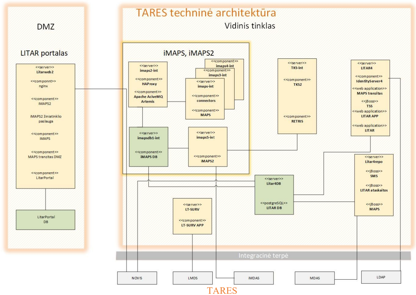
9 pav. Bendroji TARES ir LT-SMS techninė architektūra
