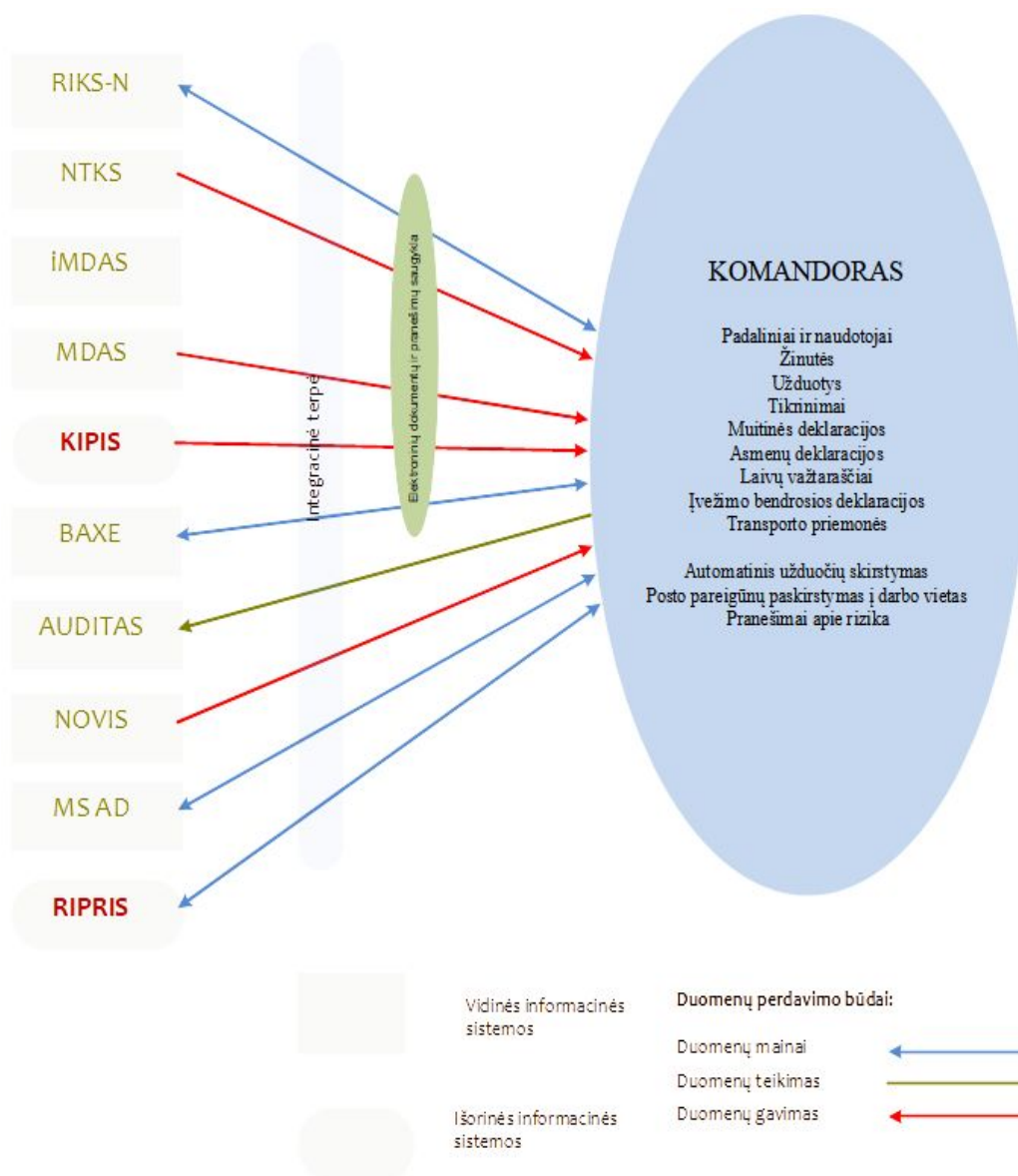
7 pav. KOMANDORAS funkcinė architektūra
