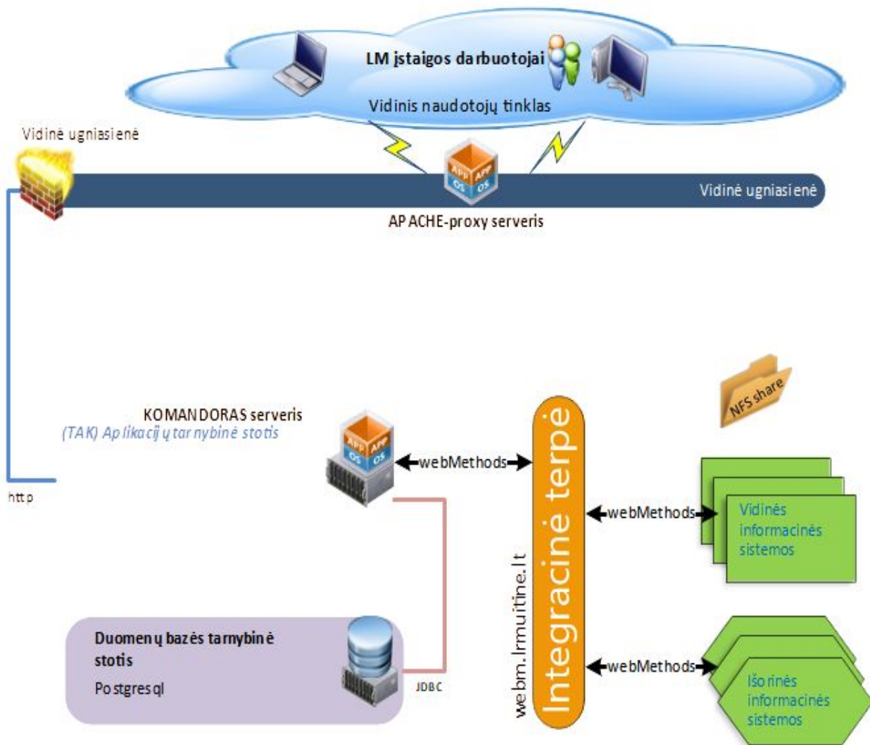
8 pav. KOMANDORAS techninė architektūra
