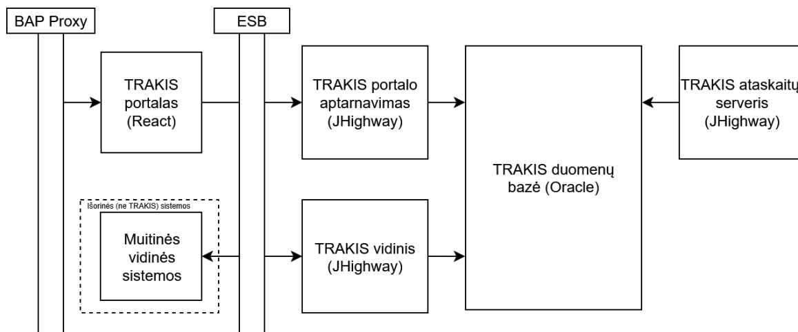
8 pav. TRAKIS architektūrinis sprendimas testavimo aplinkoje
