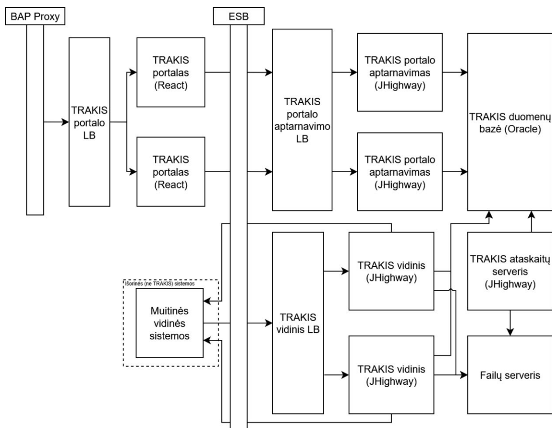
7 pav. TRAKIS architektūrinis sprendimas gamybinėje aplinkoje
