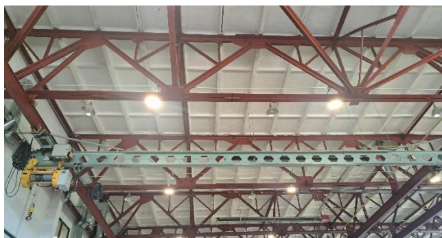
2. Pav. Viensijinis tiltinis kranas Nr. 2 3.2-15.6-15-18-400
