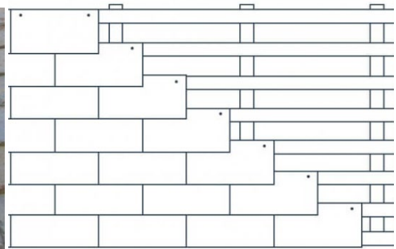
1 pav. Skalūno stogo danga ir montavimo schema
