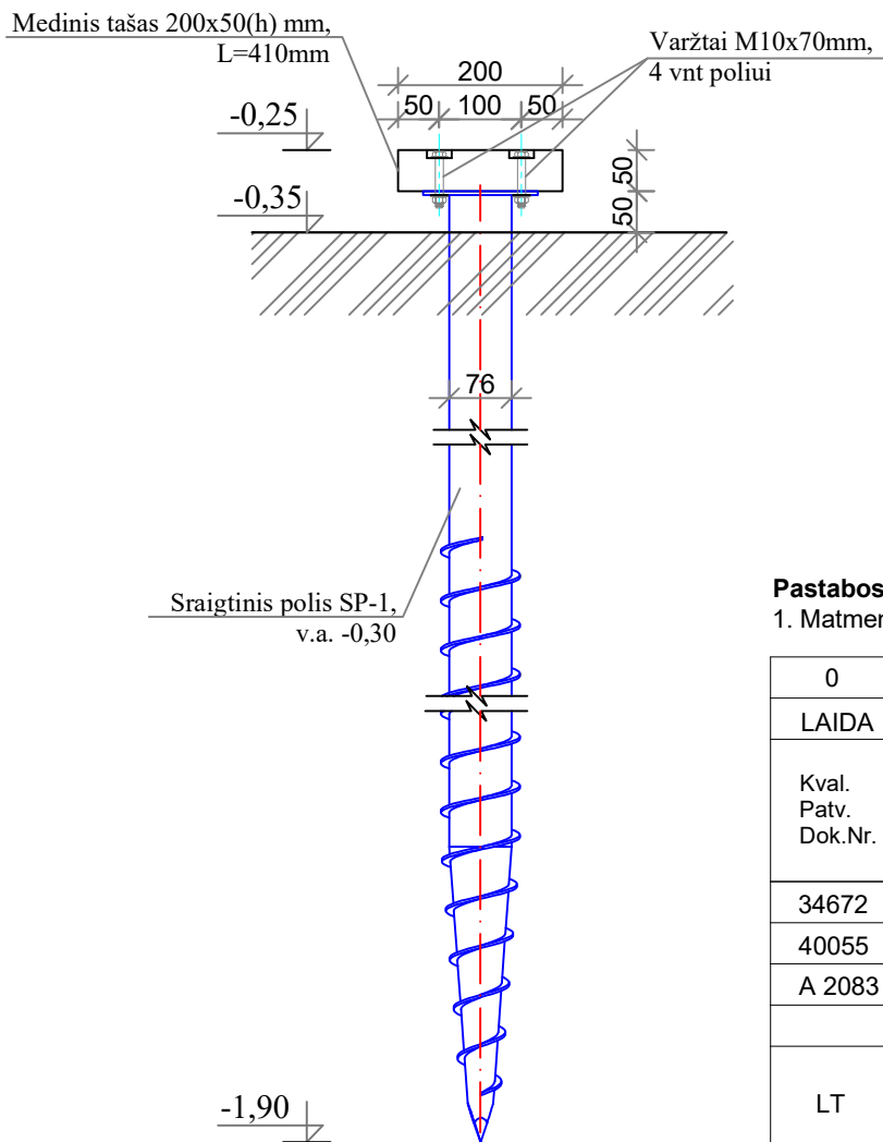
Pjūvis 2-2 M 1:10
