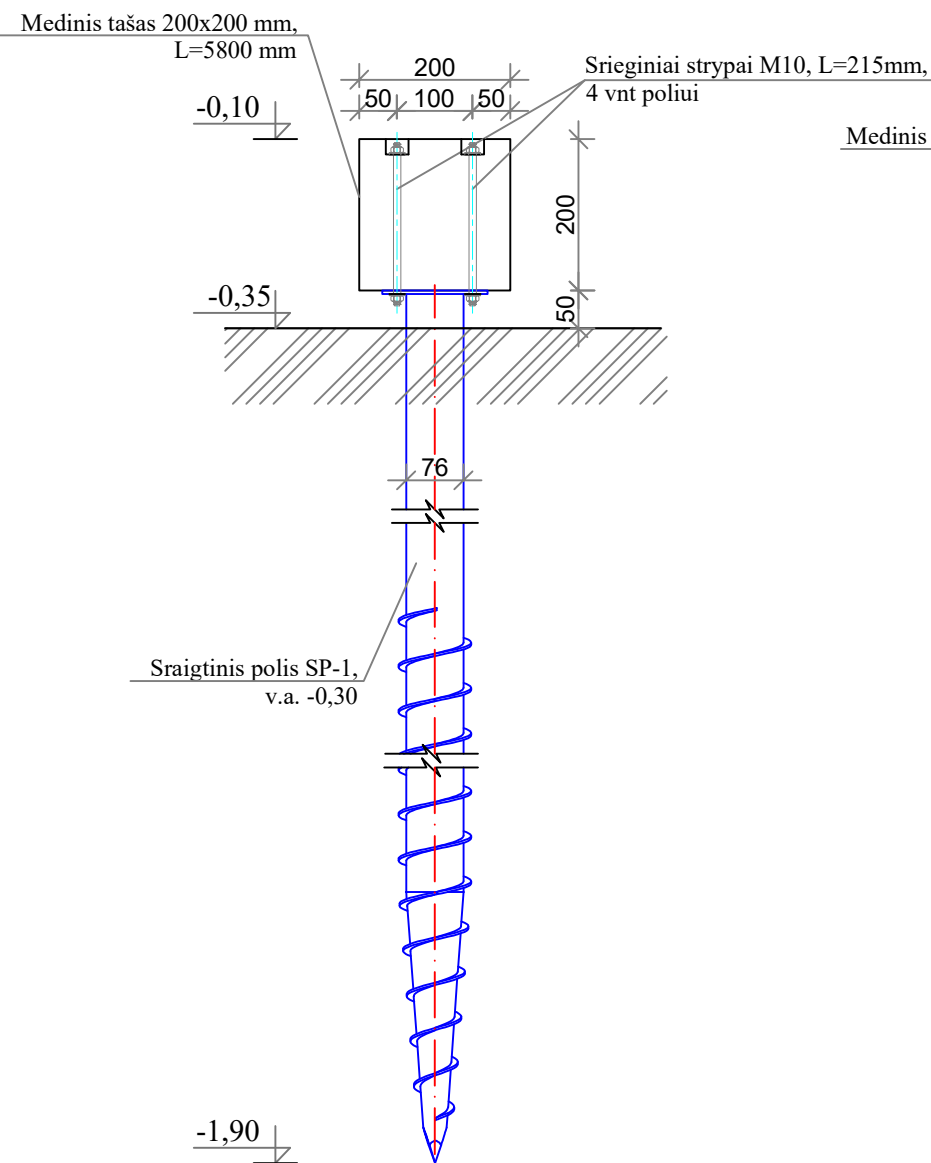
Pjūvis 1-1 M 1:10
