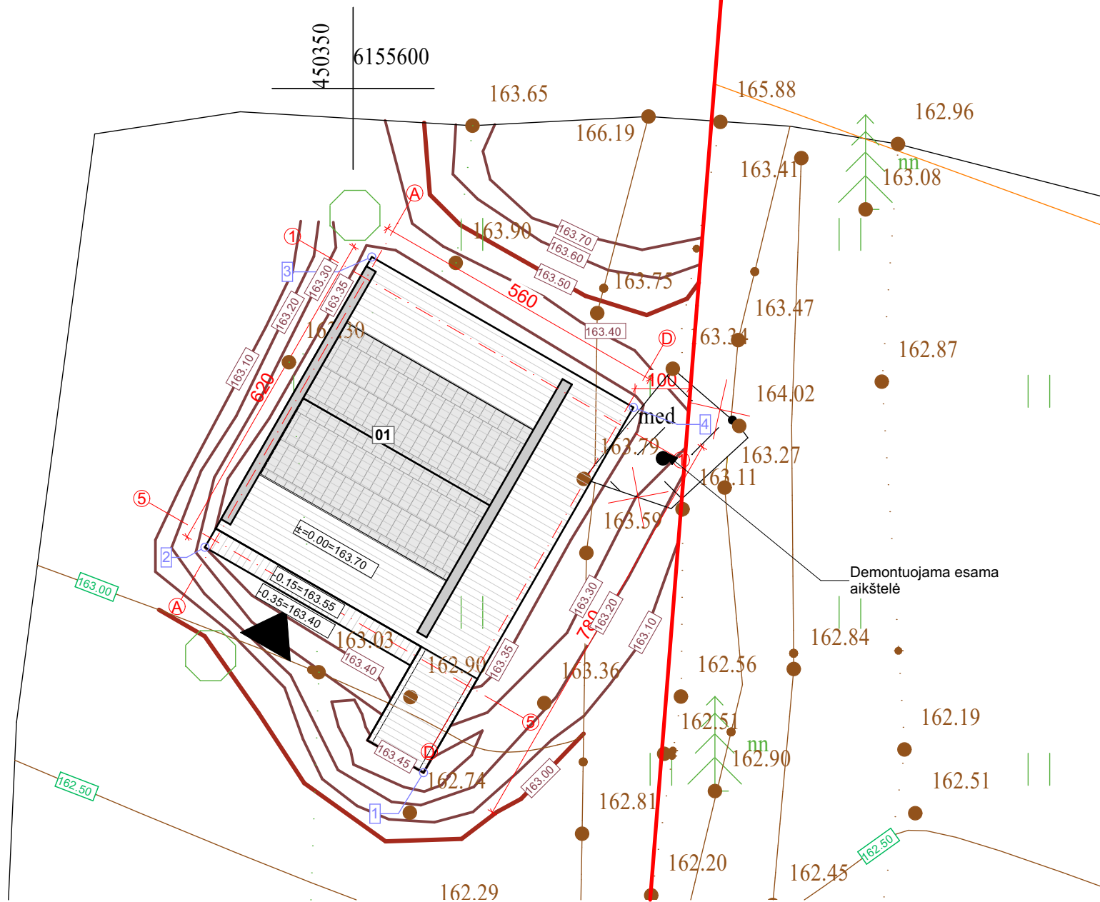
Sklypo unikalus Nr. 4400-2099-0745 vertikalus planas
