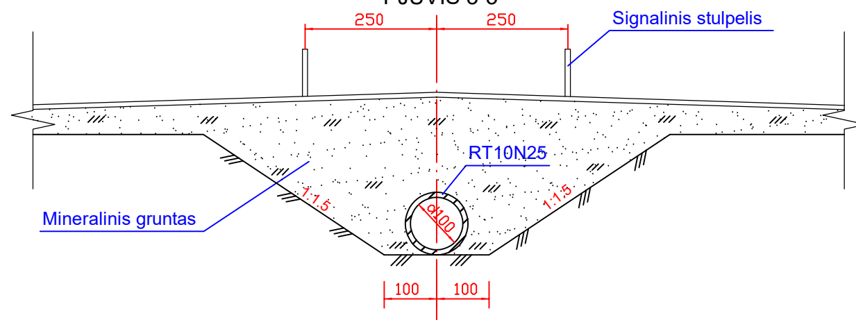
PJŪVIS 3-3
