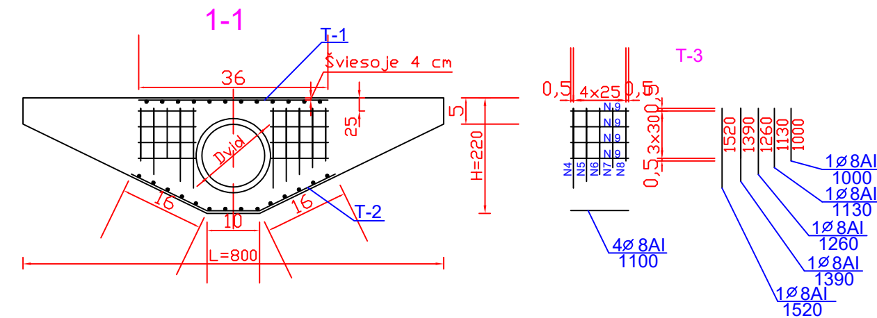
ARMATŪROS SPECIFIKACIJA
