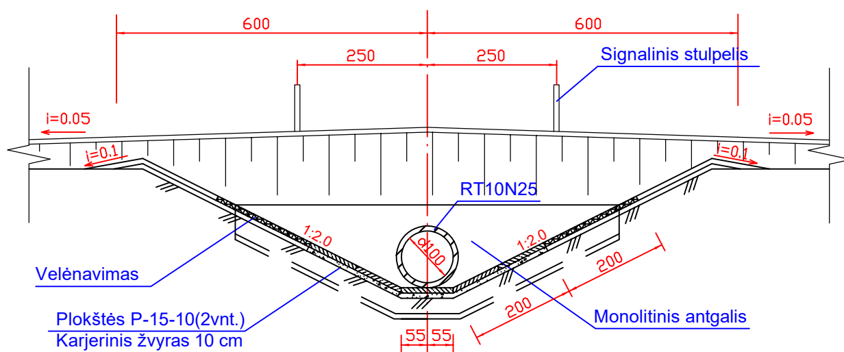
PJŪVIS 2-2
