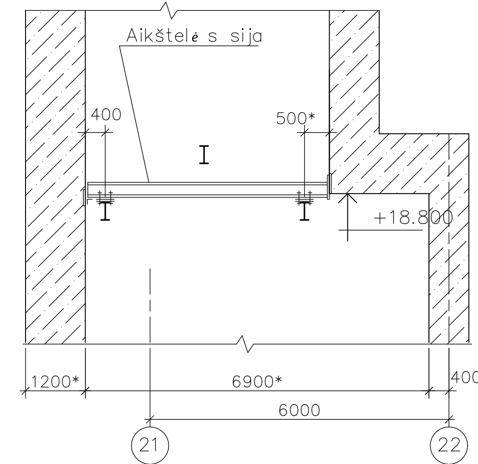
1 - 1 M 1:75 Aikštelių ir matmenys nurodyti sąlyginai
