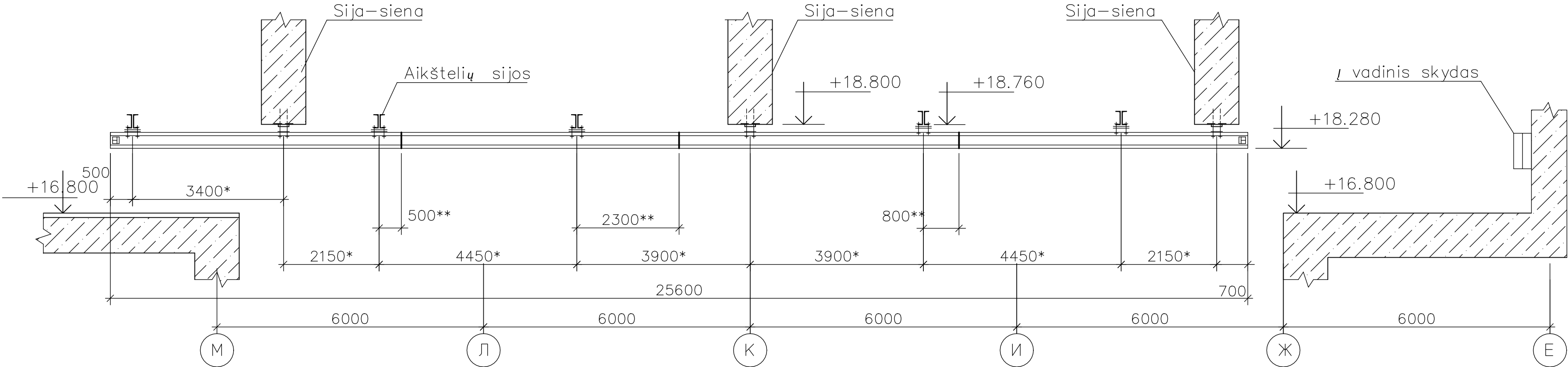
2 – 2 M 1:75 Aikštelė s ir matmenys nurodyti sąlyginai
