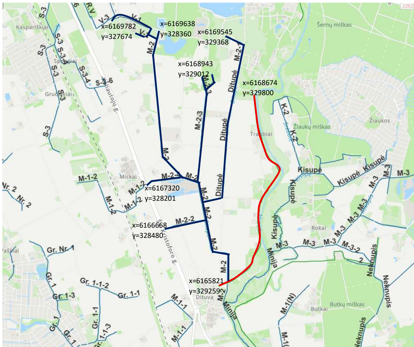
1 pav. Melioracijos statiniai Dituvos polderyje.
