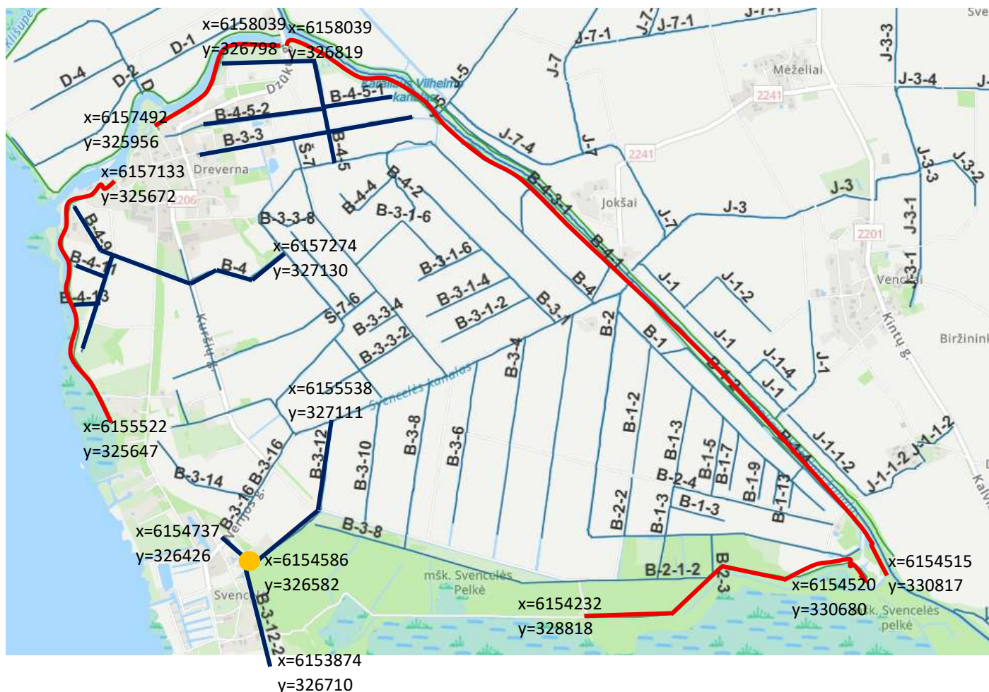
5 pav. Melioracijos statiniai Brokšvų polderyje.
