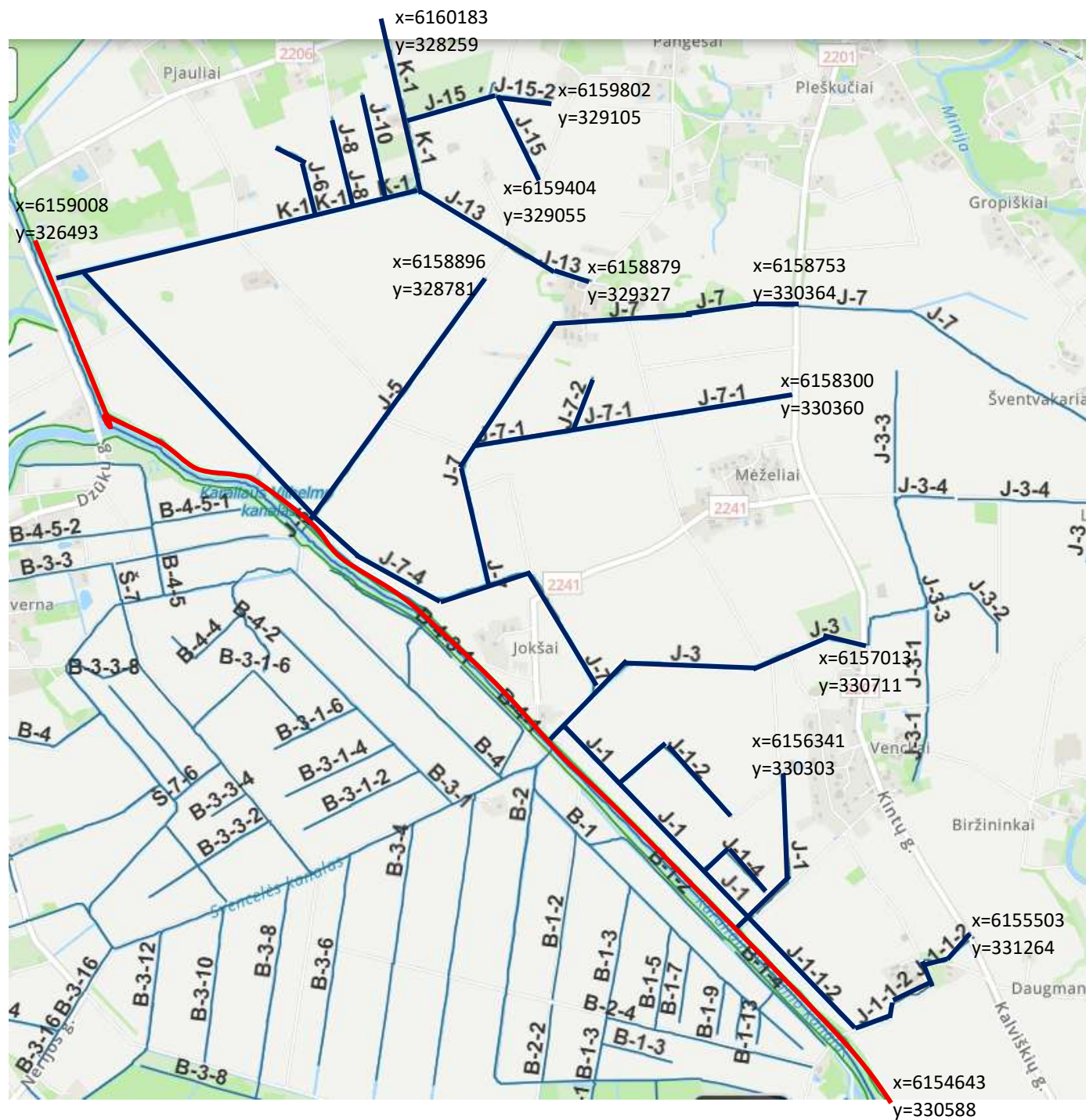
2 pav. Melioracijos statiniai Jokšų polderyje.
