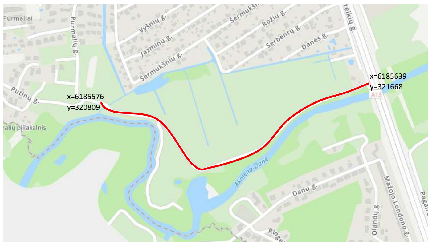
6 pav. Purmalių pylimas.
