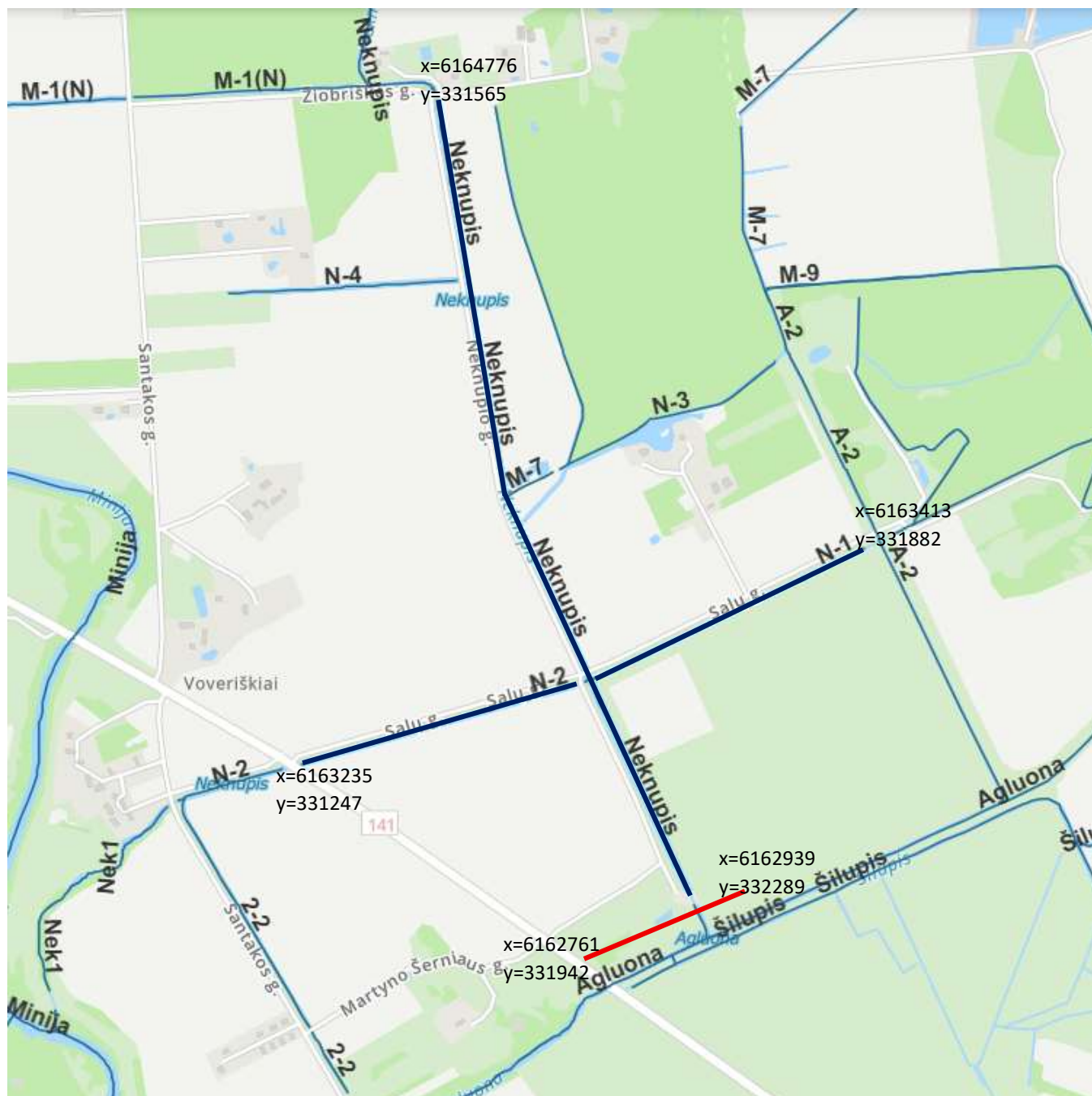
3 pav. Melioracijos statiniai Stragnų polderyje.
