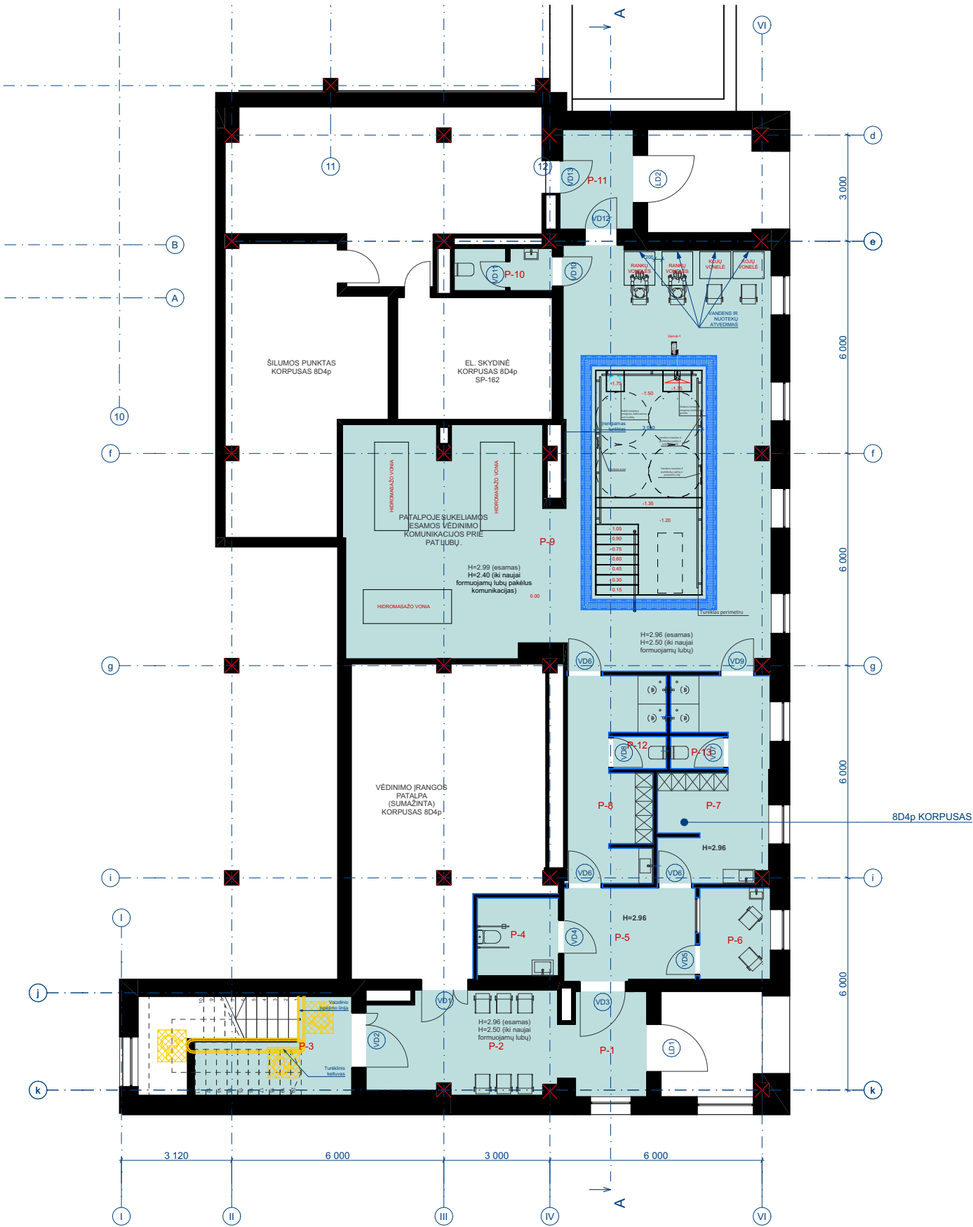
PUSRŪSIO PLANAS 1:150
