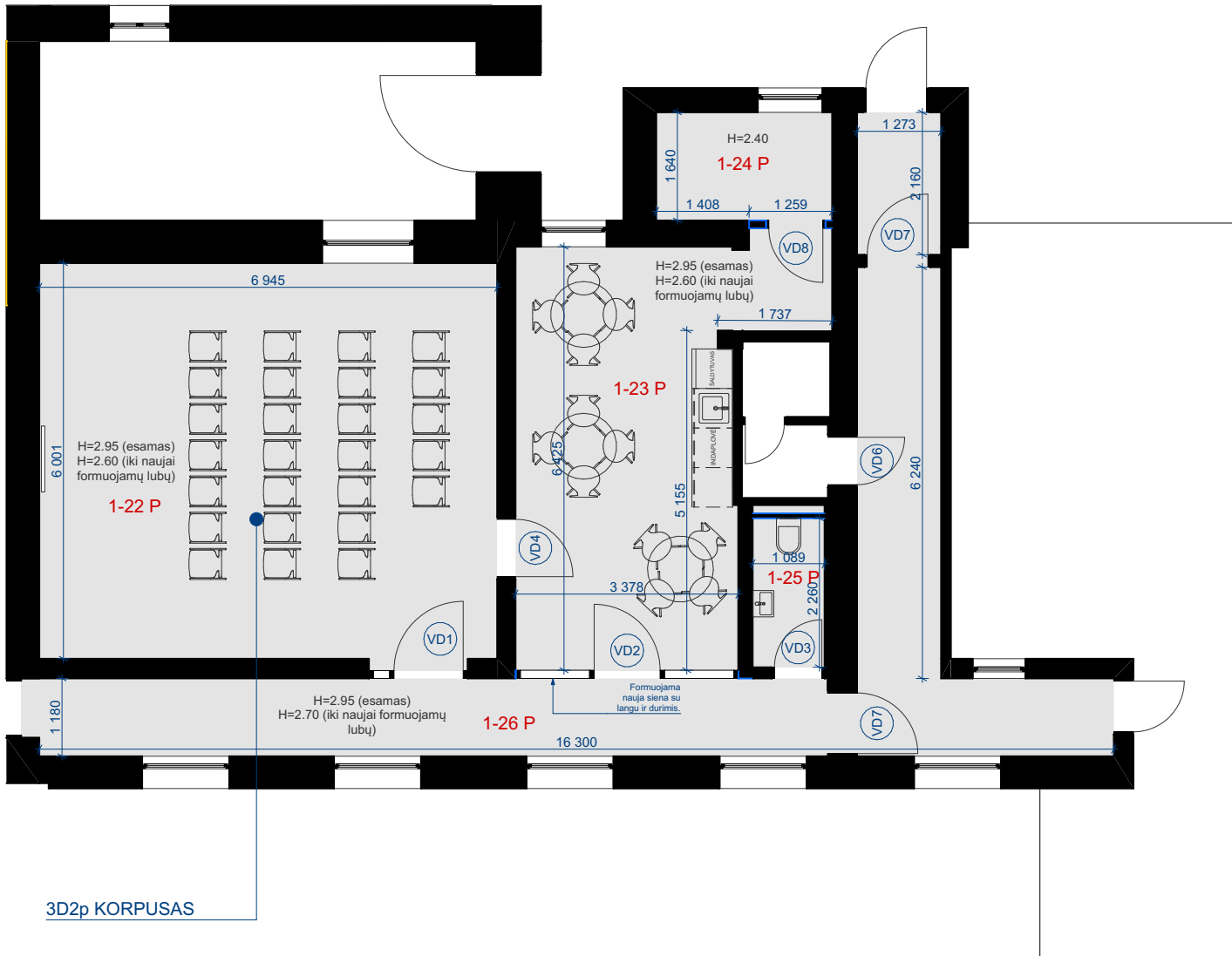
PIRMAS AUKŠTAS 1:100
