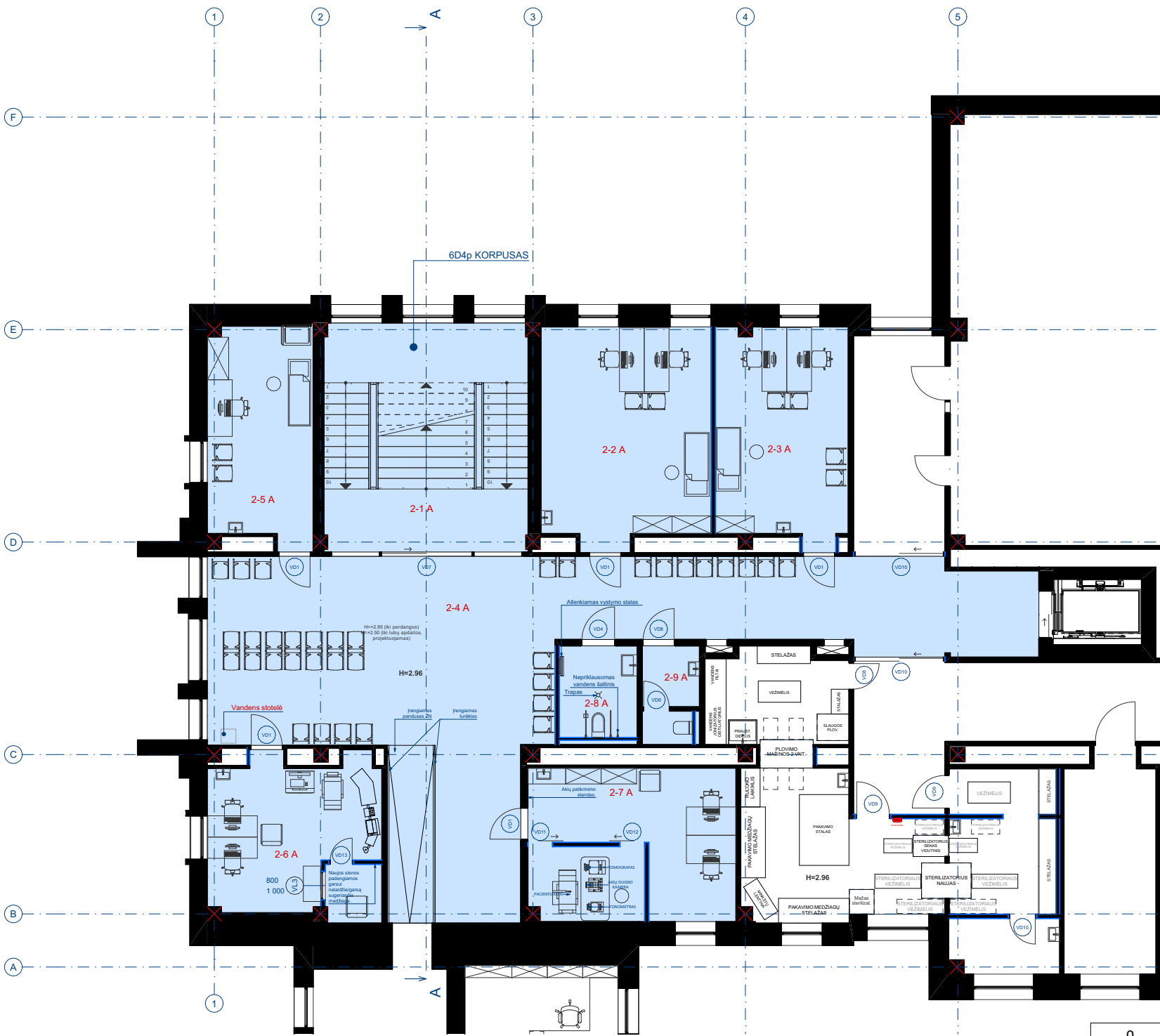
ANTRAS AUKŠTAS 1:150
