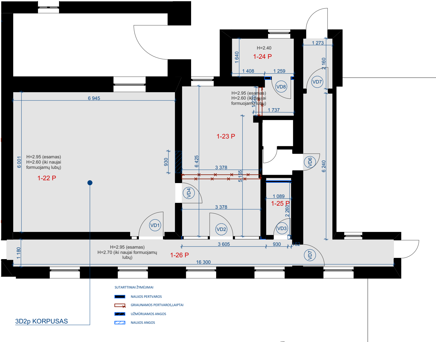
PIRMAS AUKŠTAS 1:100
