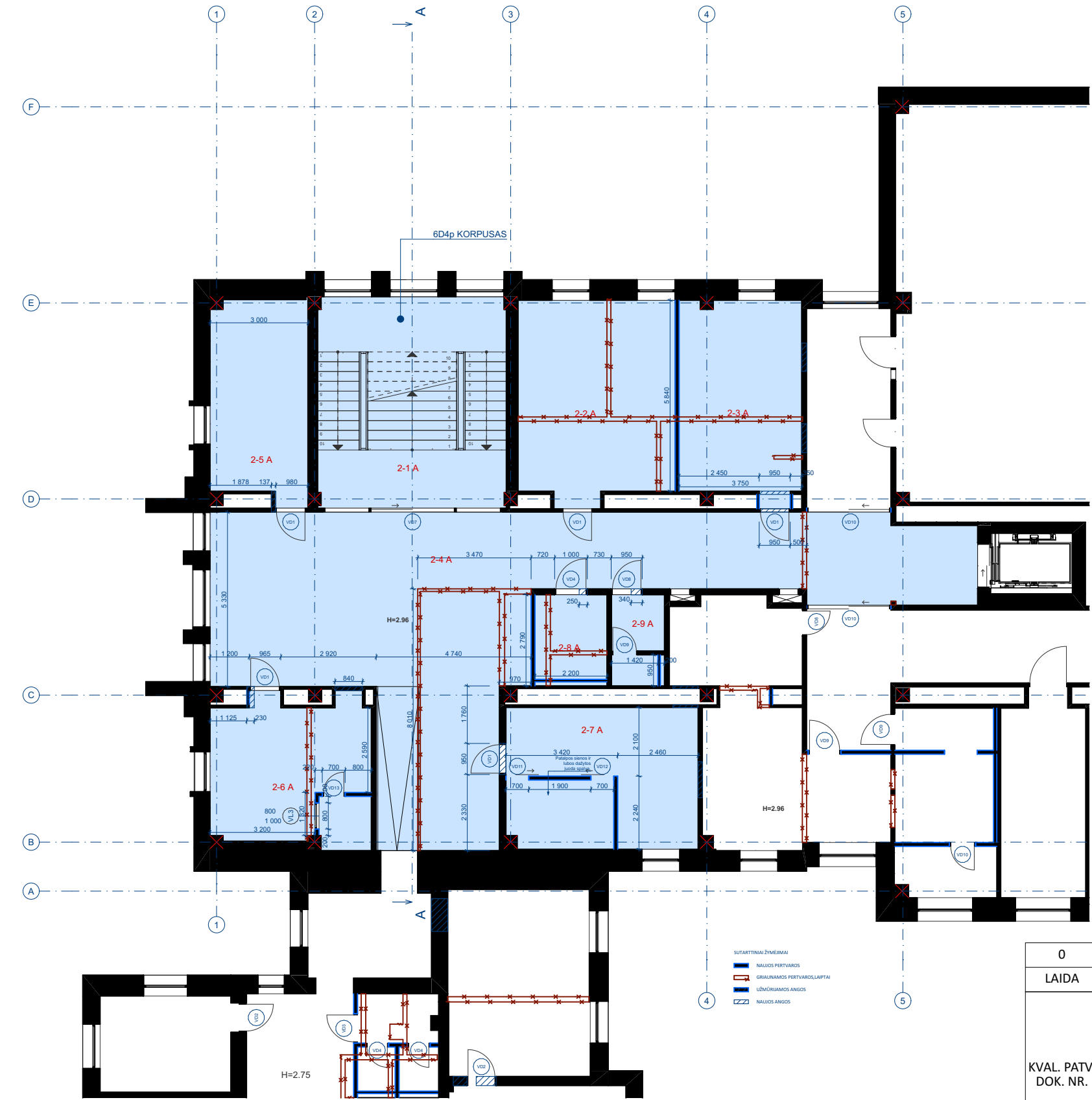
ANTRAS AUKŠTAS 1:150
