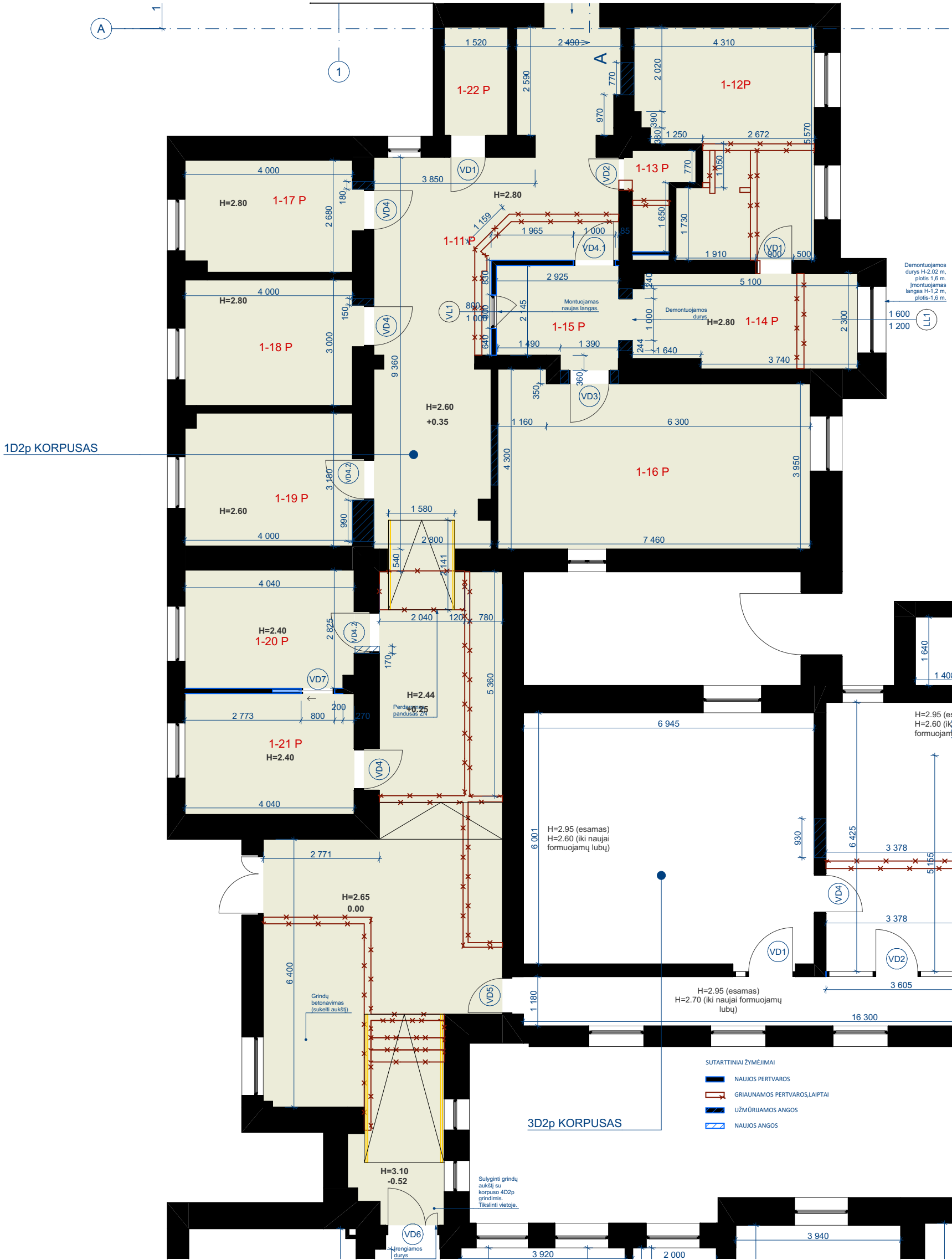
PIRMAS AUKŠTAS 1:100
