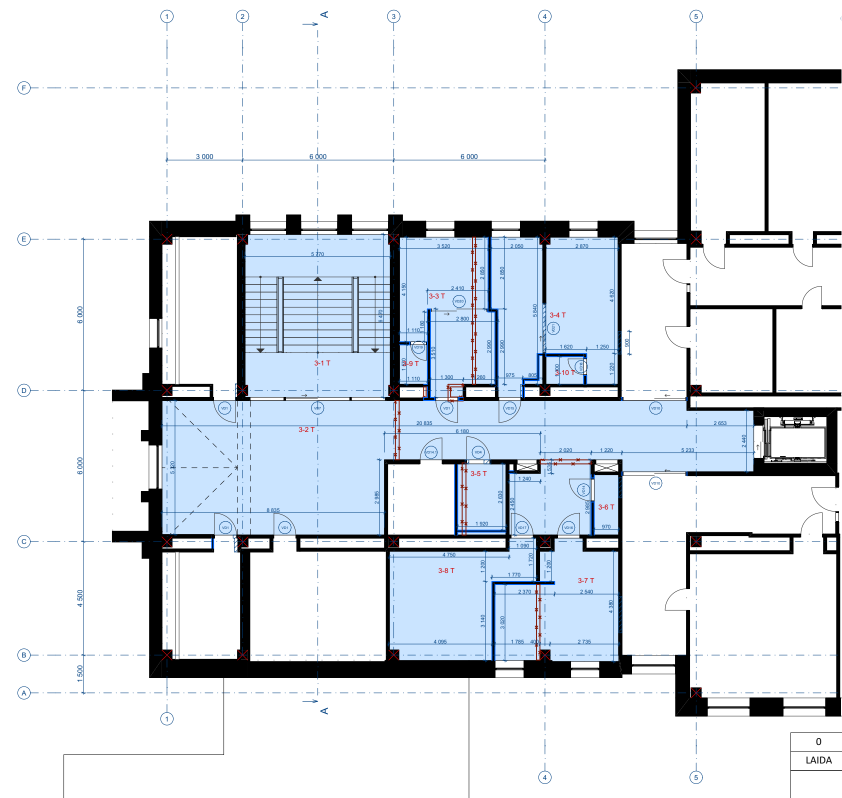
TREČIAS AUKŠTAS 1:150
