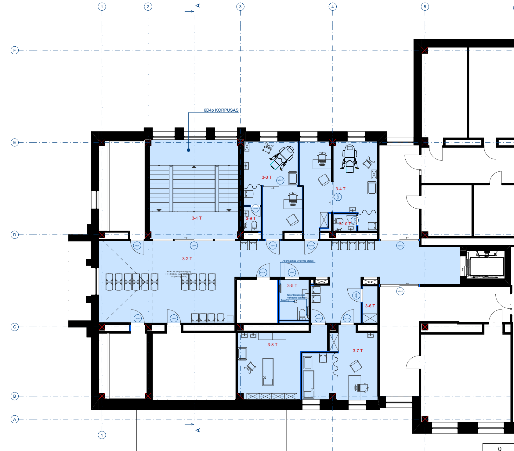
3. TREČIAS AUKŠTAS 1:150
