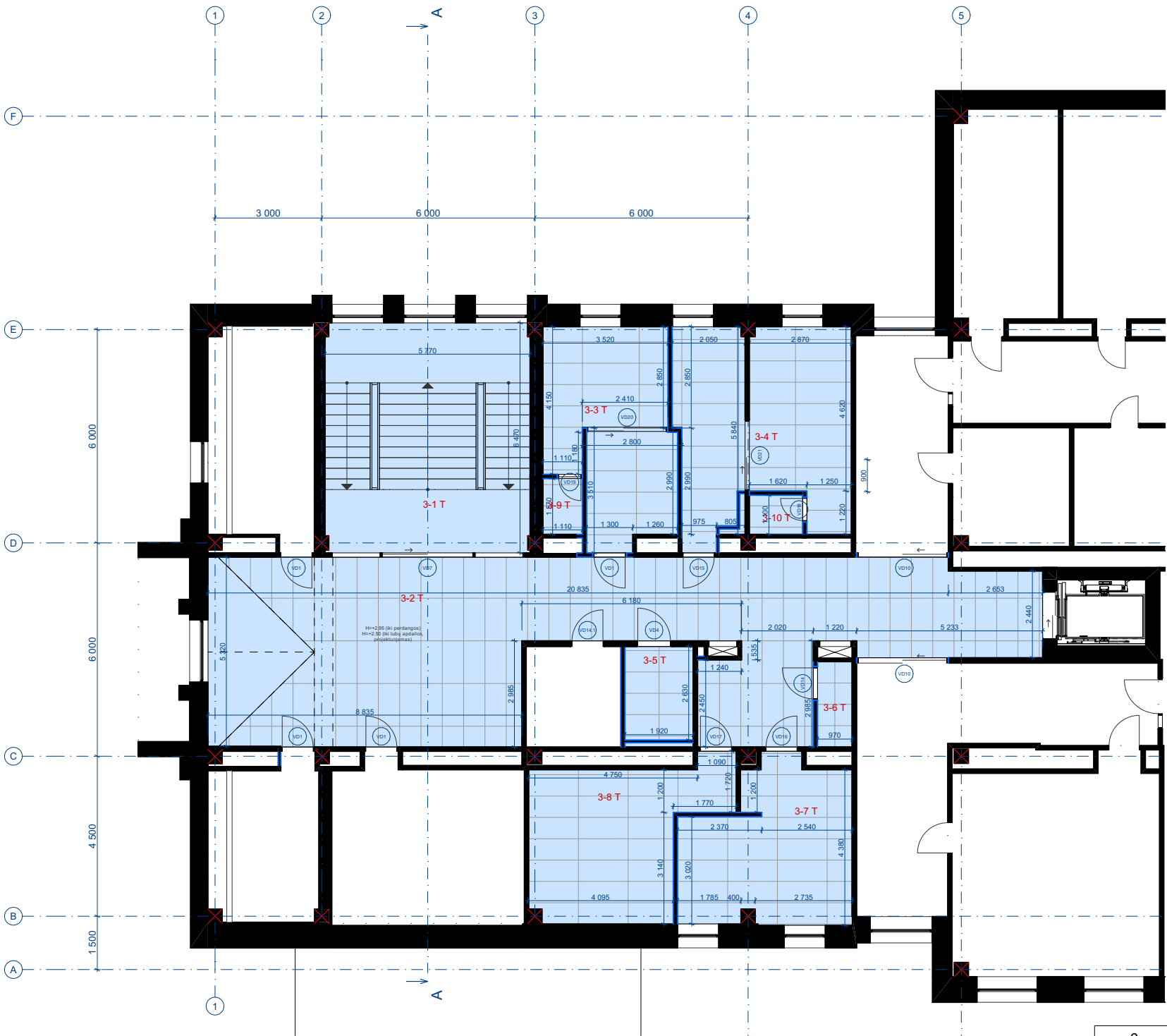
TREČIAS AUKŠTAS 1:150
