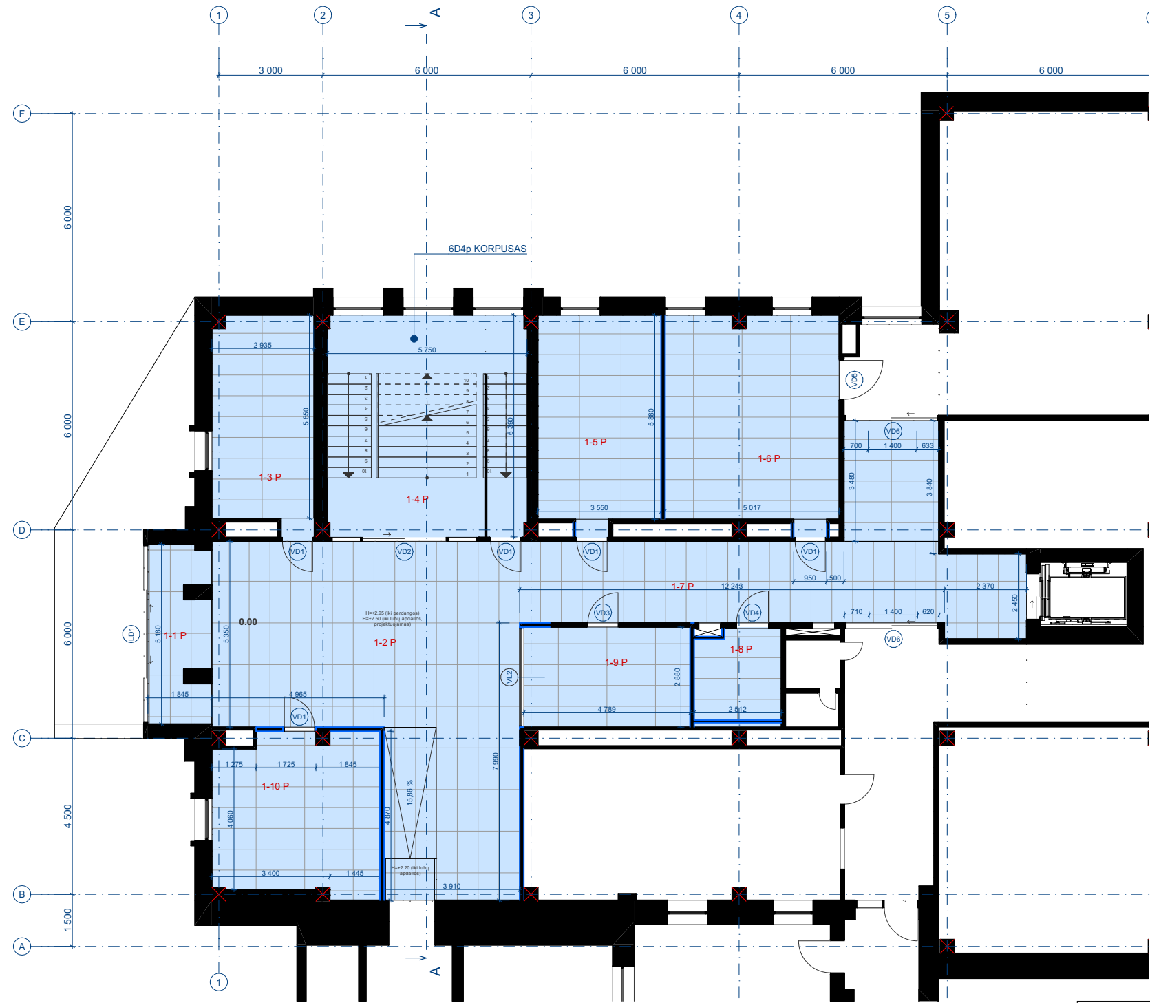
PIRMAS AUKŠTAS 1:150
