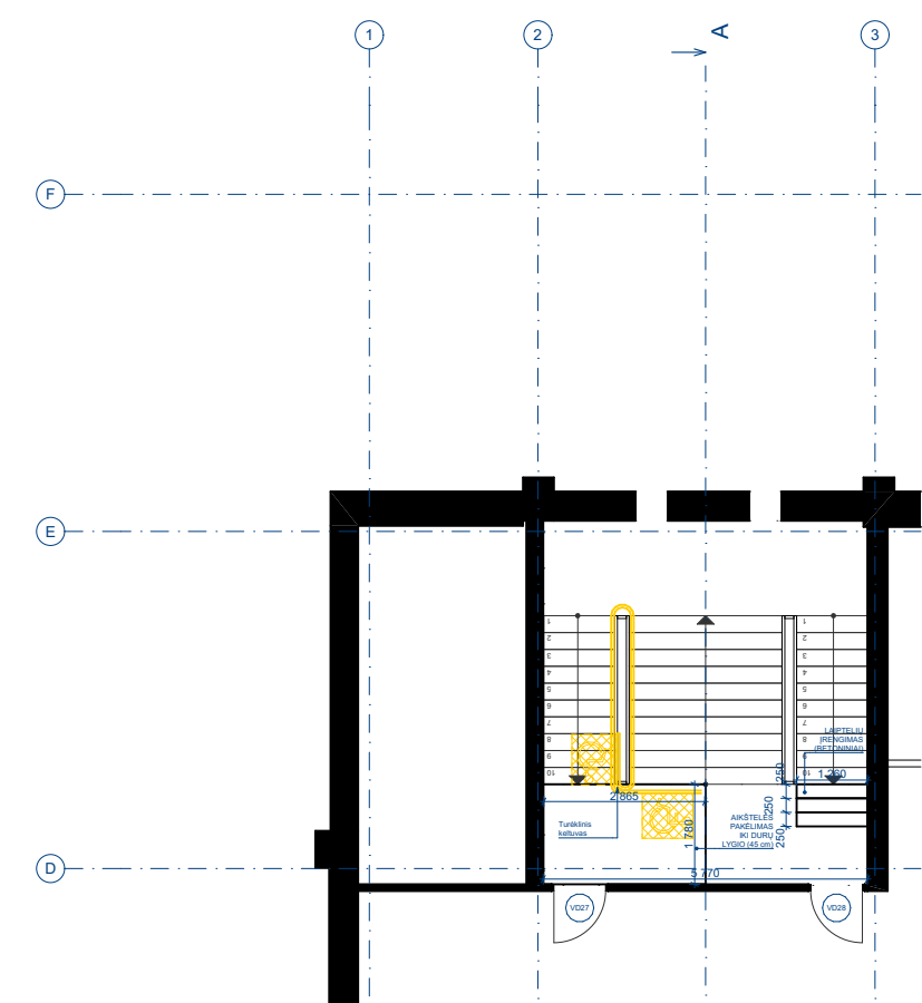
TECHNINIS AUKŠTAS 1:150
