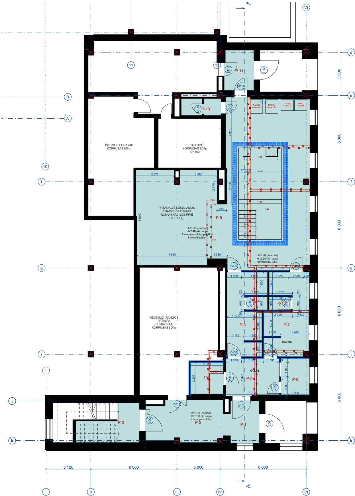
PUŠRŪSIO PLANAS 1:150
