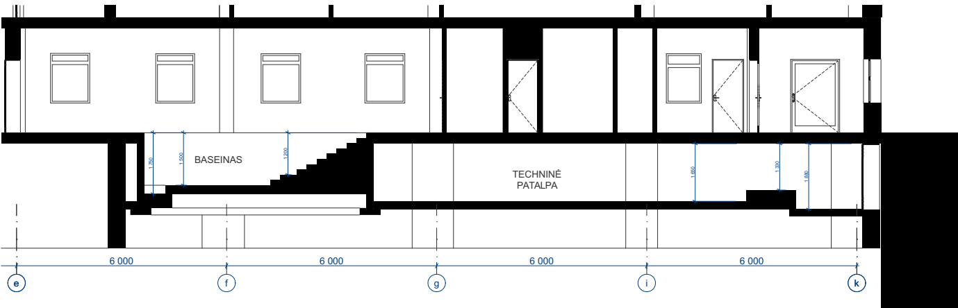
BASEINO PJŪVIS 1:150
