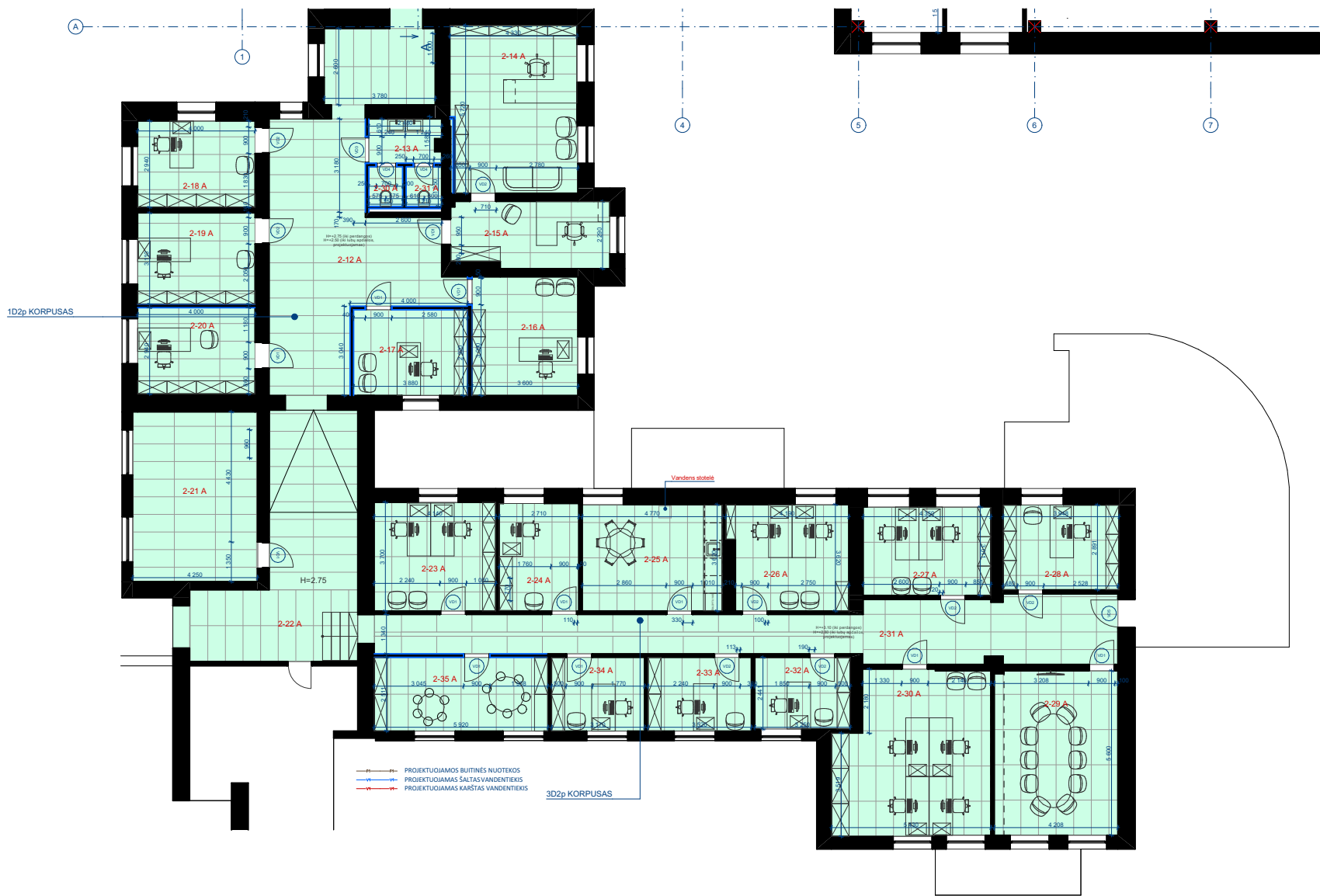
ANTRAS AUKŠTAS
