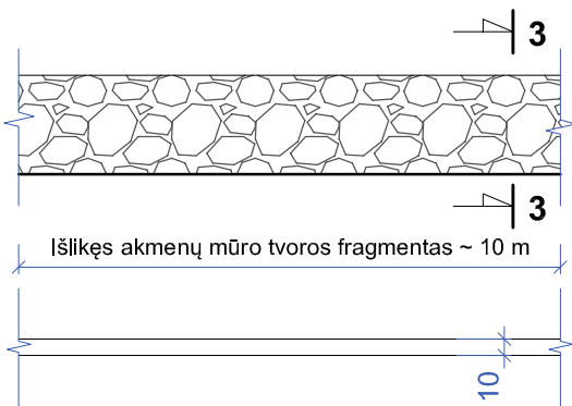
PLANAS M 1:50
