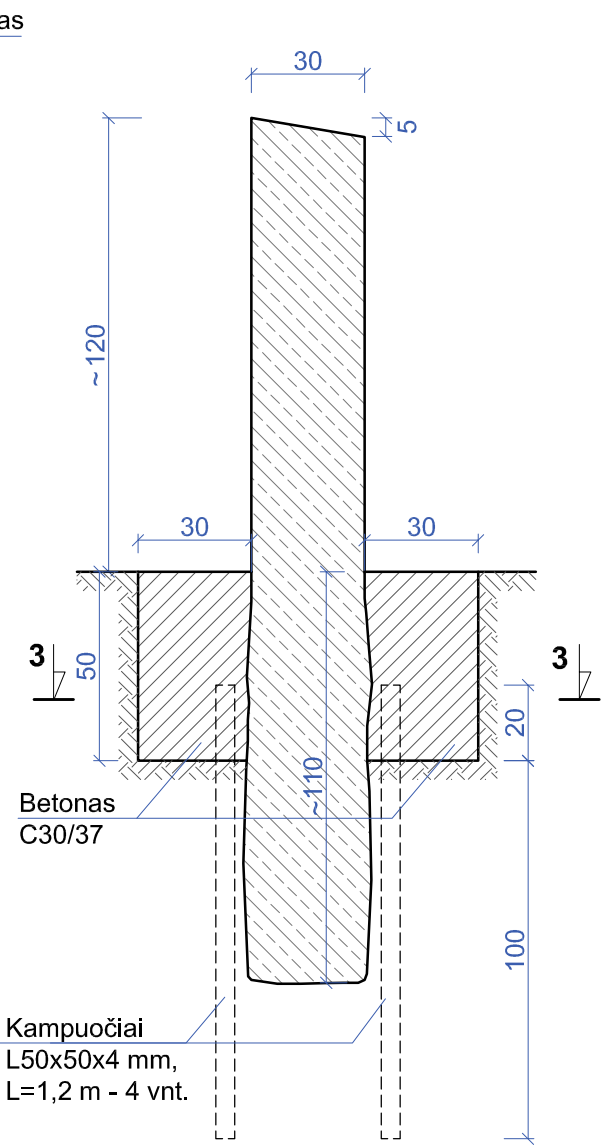
2-2 M 1:20
