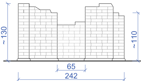
VAIZDAS A-A M 1:50
