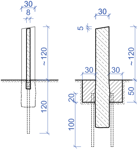
1-1 M 1:50
