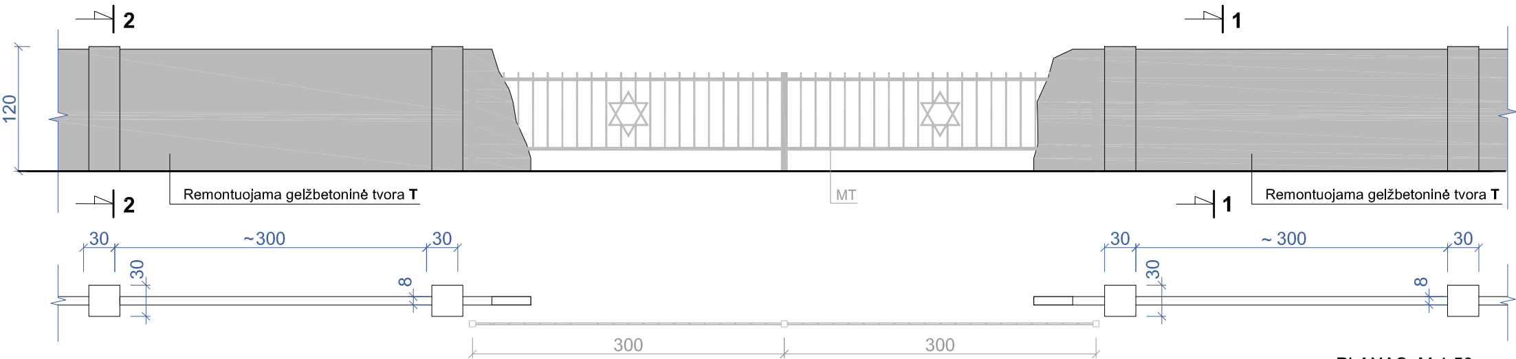
GELŽBETONINĖS TVOROS T FRAGMENTAS PR PUSĖJE. VAIZDAS IŠ PRIEKIO M 1:50
